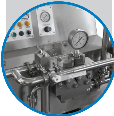
Detalles homogenizador/ Detalhe do cabeçote de homogeneização
