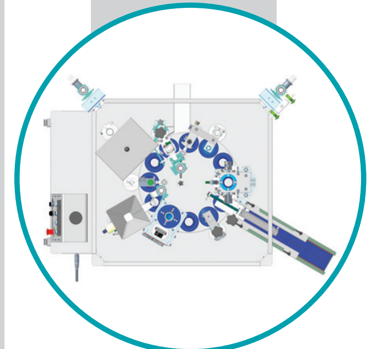
Vista total de la máquina/ Visão total da máquina
