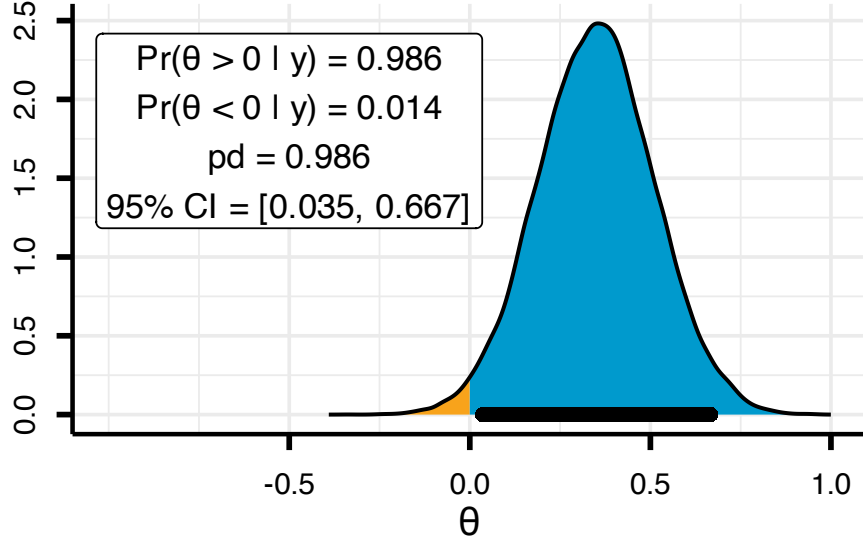
Posterior density
