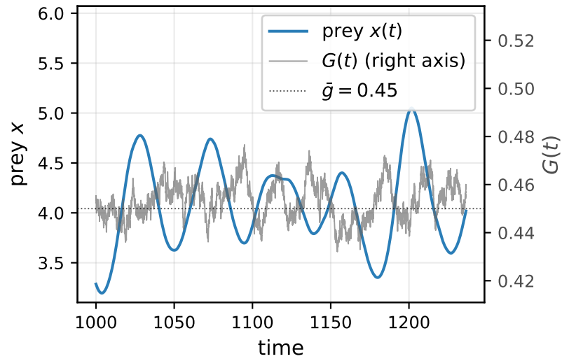
(d) \alpha = 0.133 , \sigma_U = 0.0182 -- resonance ( \tau_{OU} = T_0/(2\pi) )
