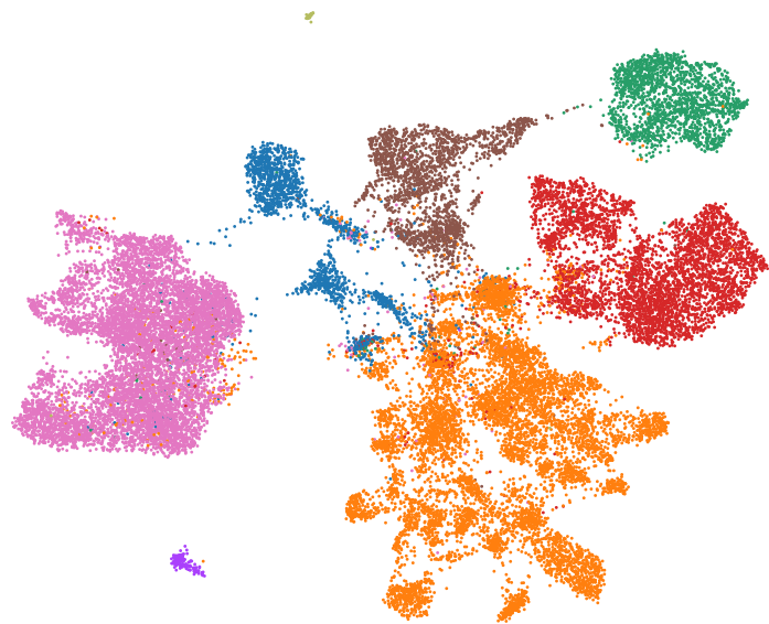
scVI
