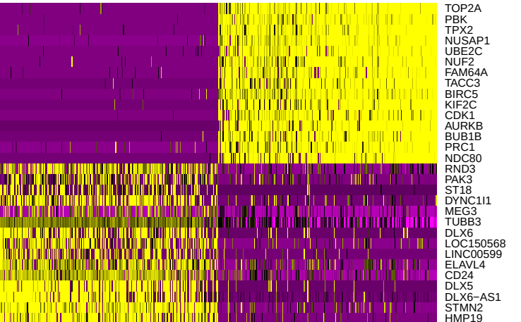
PC_2
