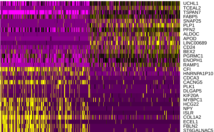
PC_7
