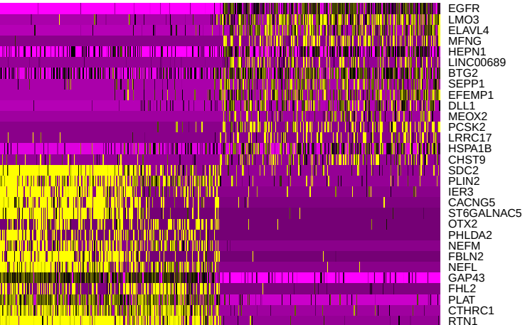
PC_5
