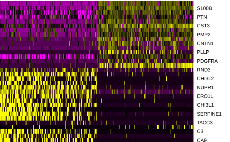
PC_4
