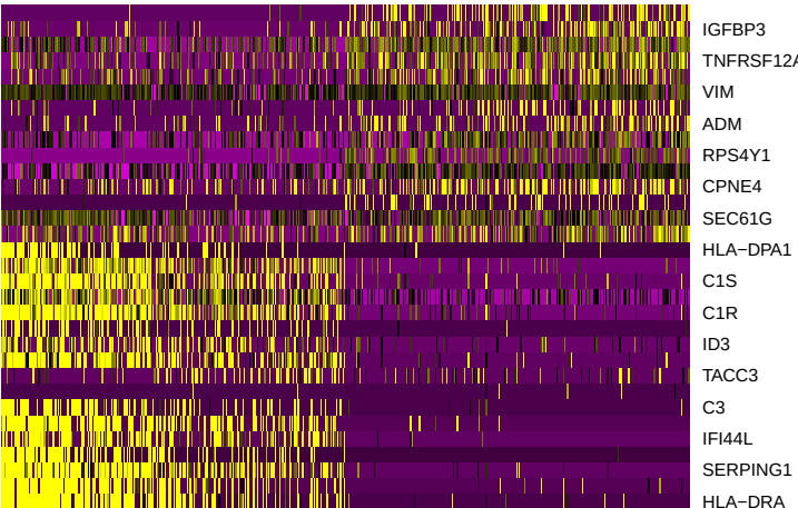
PC_9
