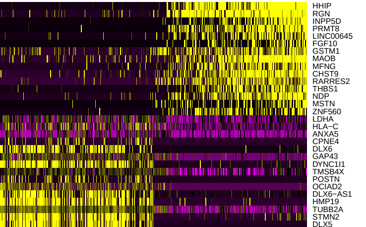
PC_8
