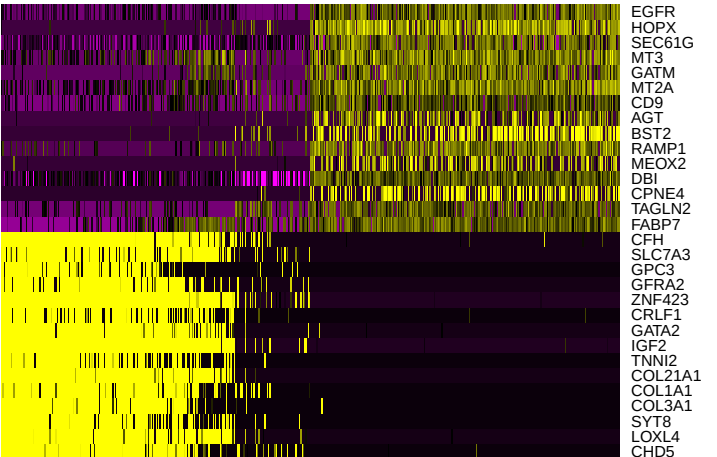
PC_3
