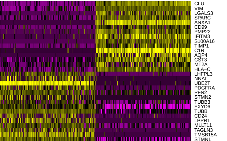
PC_1
