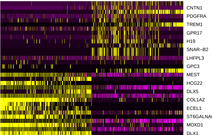
PC_6
