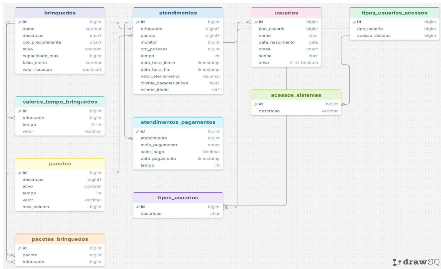
Figura 1 — Diagrama ER do Sistema ServioKids (drawSQL)
