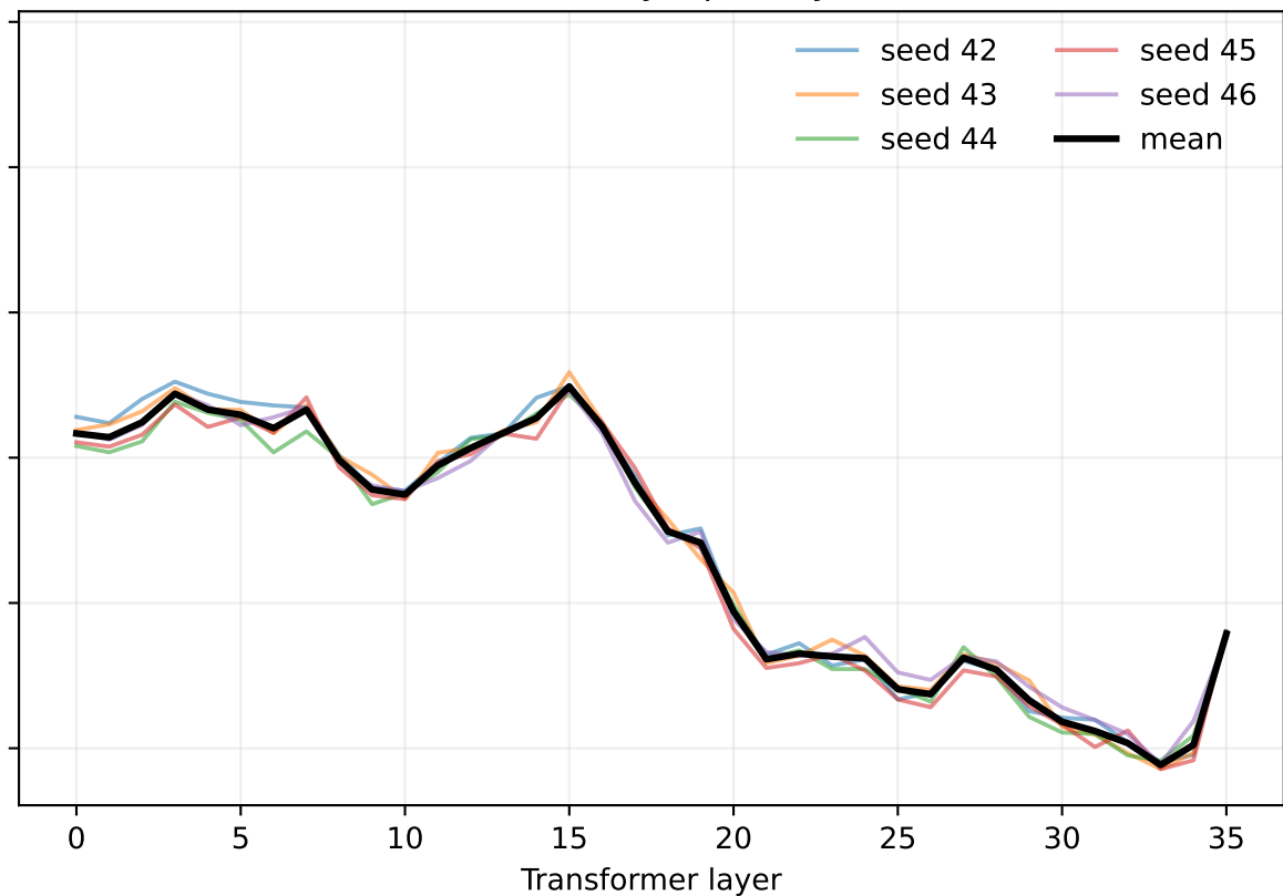
NS: non-sycophancy
