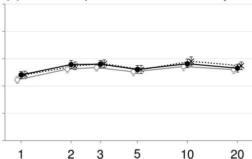
(d) Hosts compromised, service diversity
