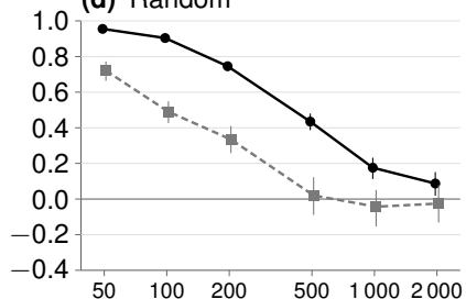
(d) Random
