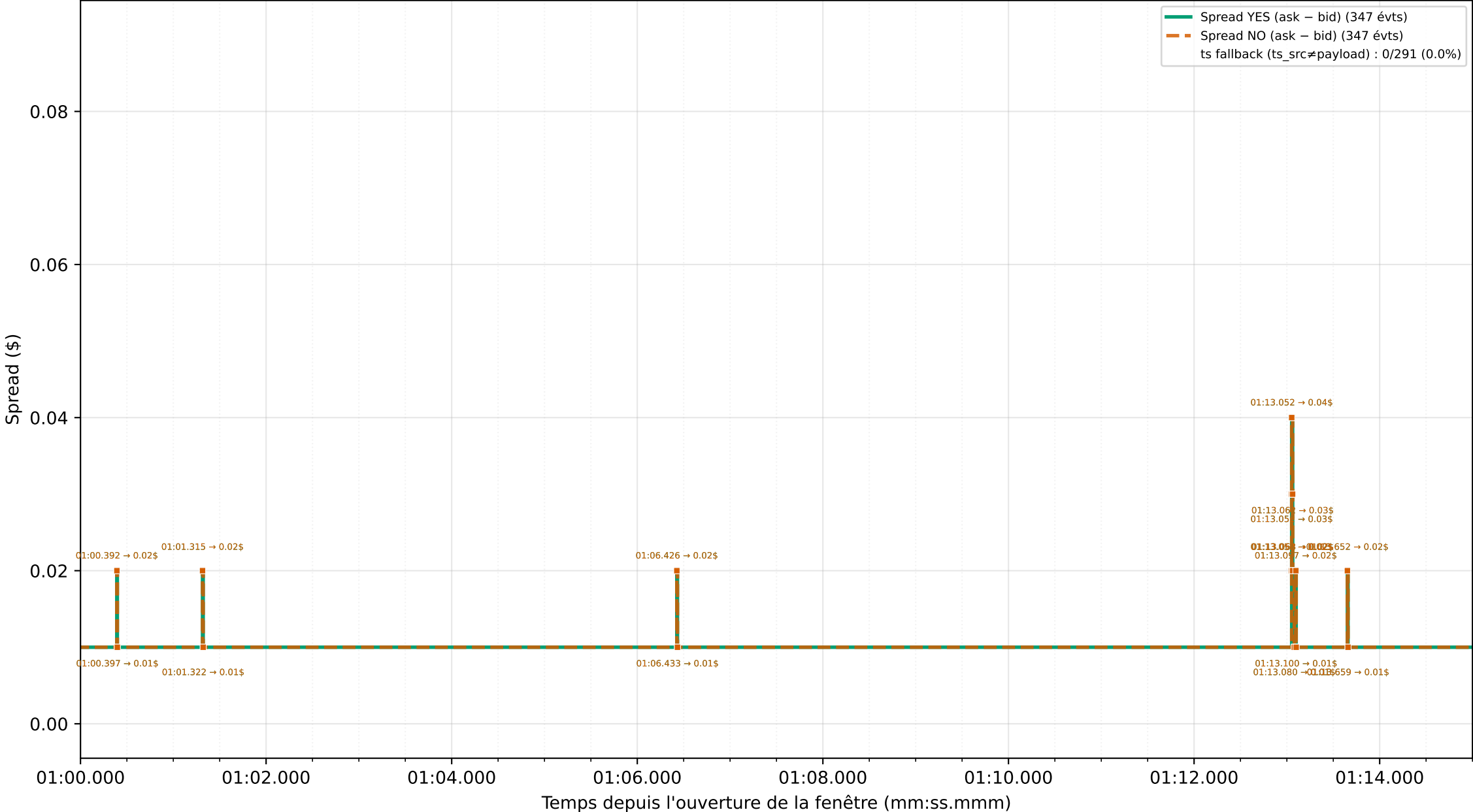
Graphique 5 : Spreads YES et NO absolus (événementiels) — zoom 15 s [01:00.000 → 01:15.000]
