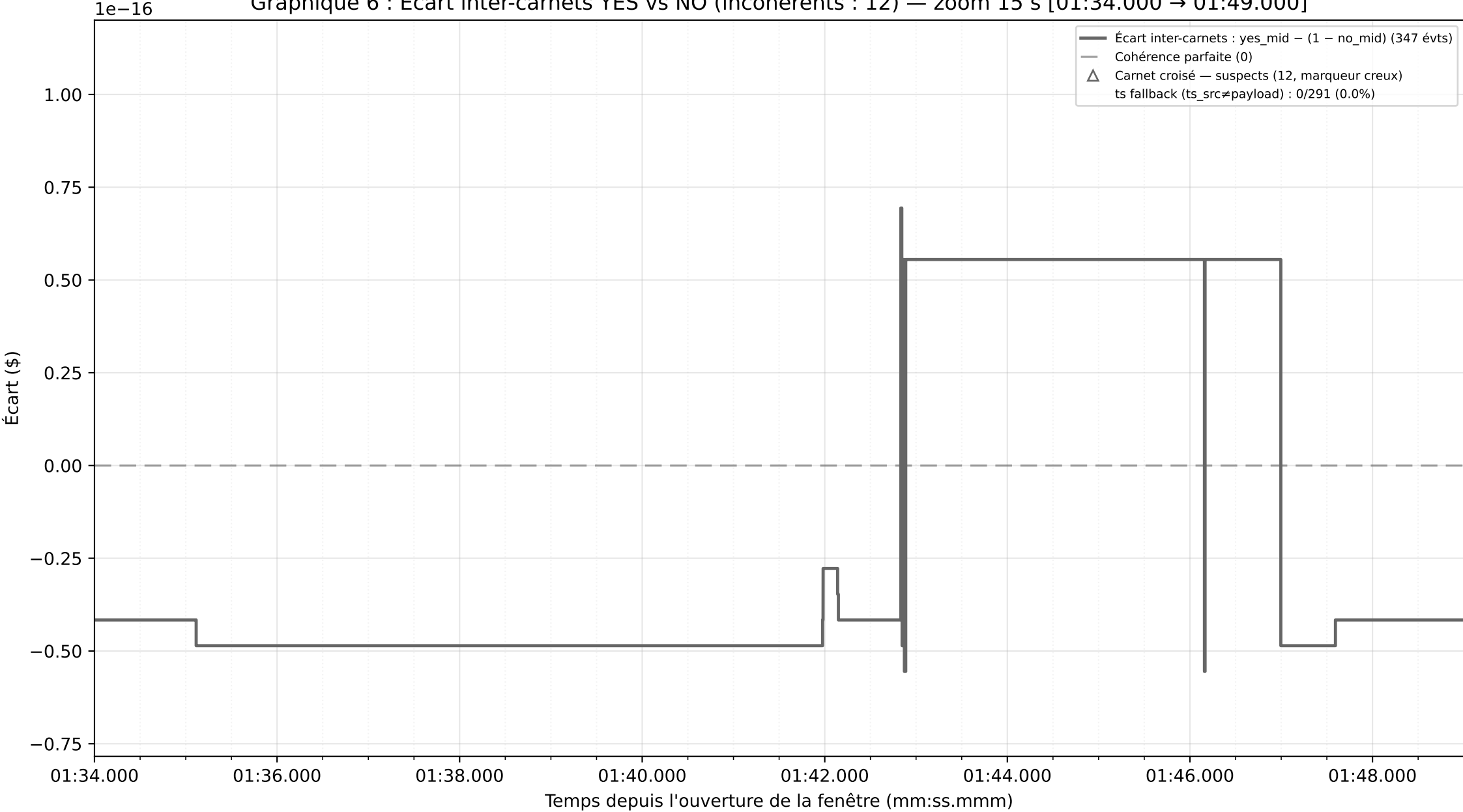
Graphique 6 : Écart inter-carnets YES vs NO (incohérents : 12) — zoom 15 s [01:34.000 → 01:49.000]
