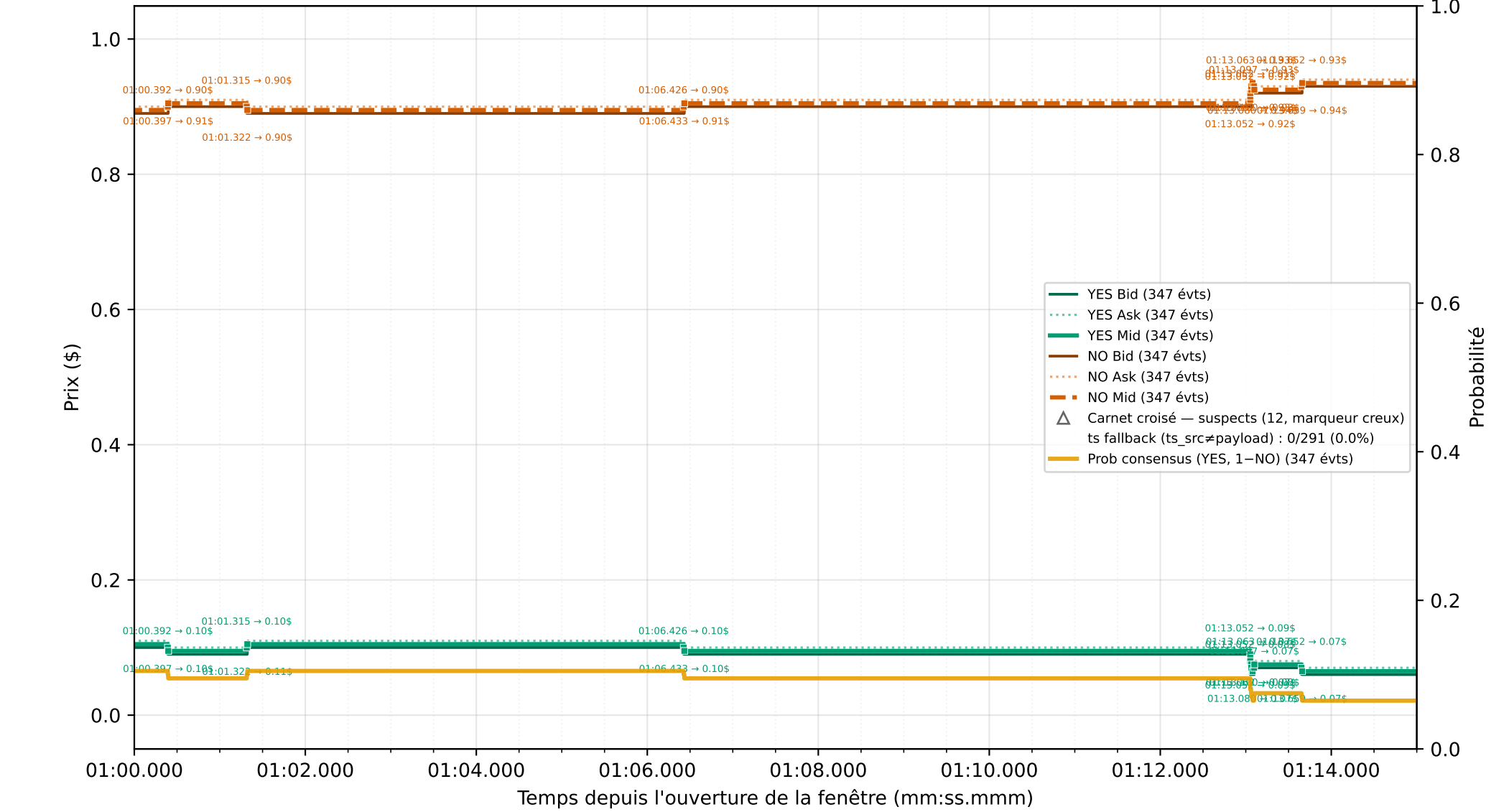
Polymarket BTC 5min | Bitcoin Up or Down - August 18, 9:00AM-9:05AM ET | Résultat : ▼ DOWN Graphique 1 : Carnet YES/NO complet — 347 événements BBO (précision ms) | incohérents : 12 — zoom 15 s [01:00.000 → 01:15.000]
