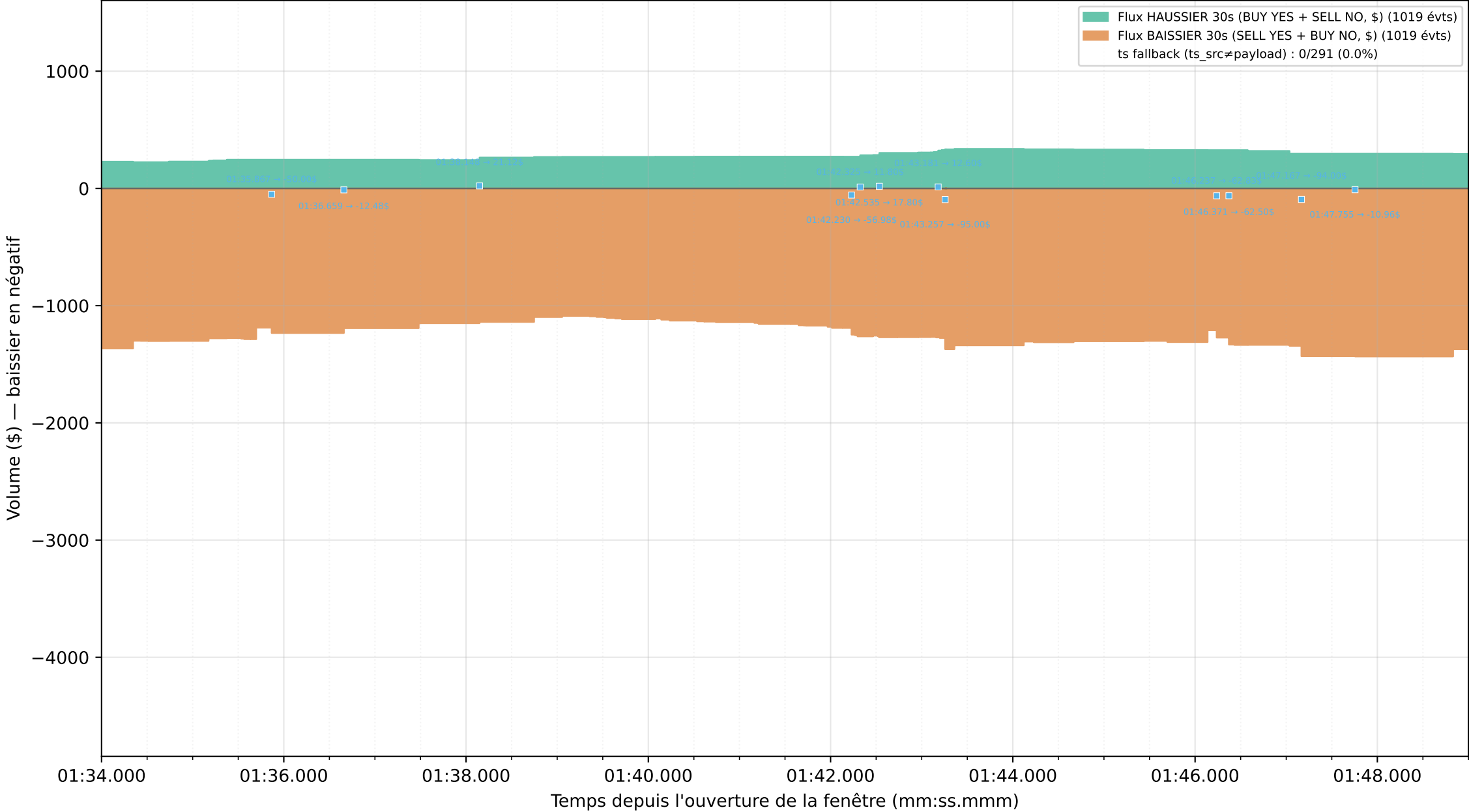
Graphique 3 : Flux directionnel normalisé YES/NO (1019 trades) — zoom 15 s [01:34.000 → 01:49.000]
