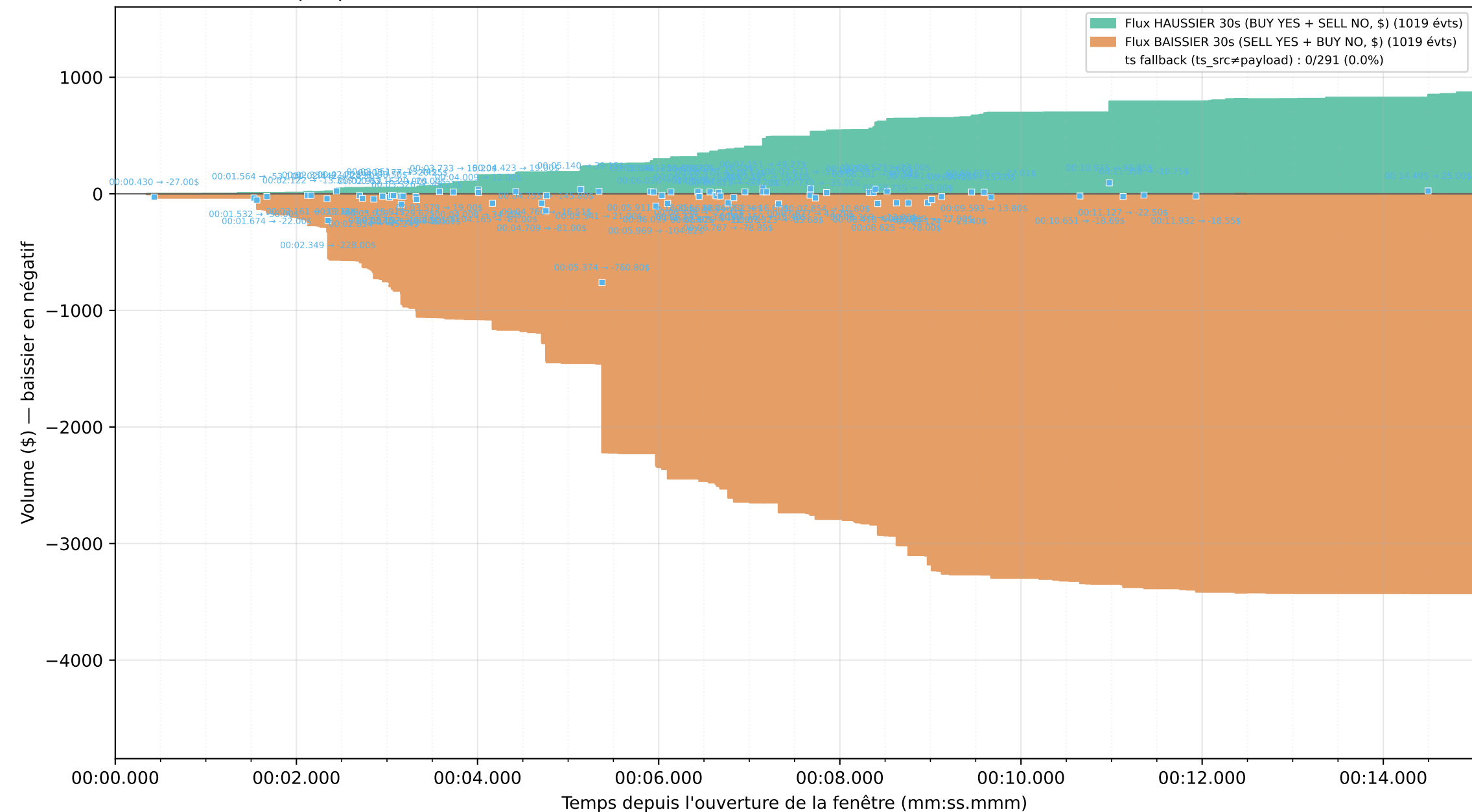
Graphique 3 : Flux directionnel normalisé YES/NO (1019 trades) — zoom 15 s [00:00.000 → 00:15.000]
