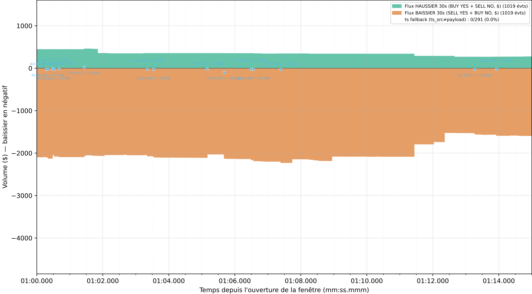
Graphique 3 : Flux directionnel normalisé YES/NO (1019 trades) — zoom 15 s [01:00.000 → 01:15.000]
