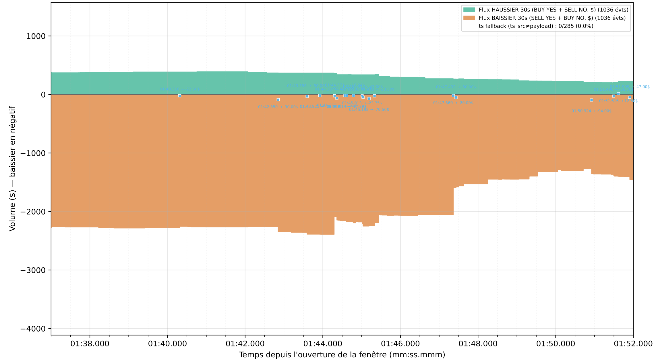
Graphique 3 : Flux directionnel normalisé YES/NO (1036 trades) — zoom 15 s [01:37.000 → 01:52.000]
