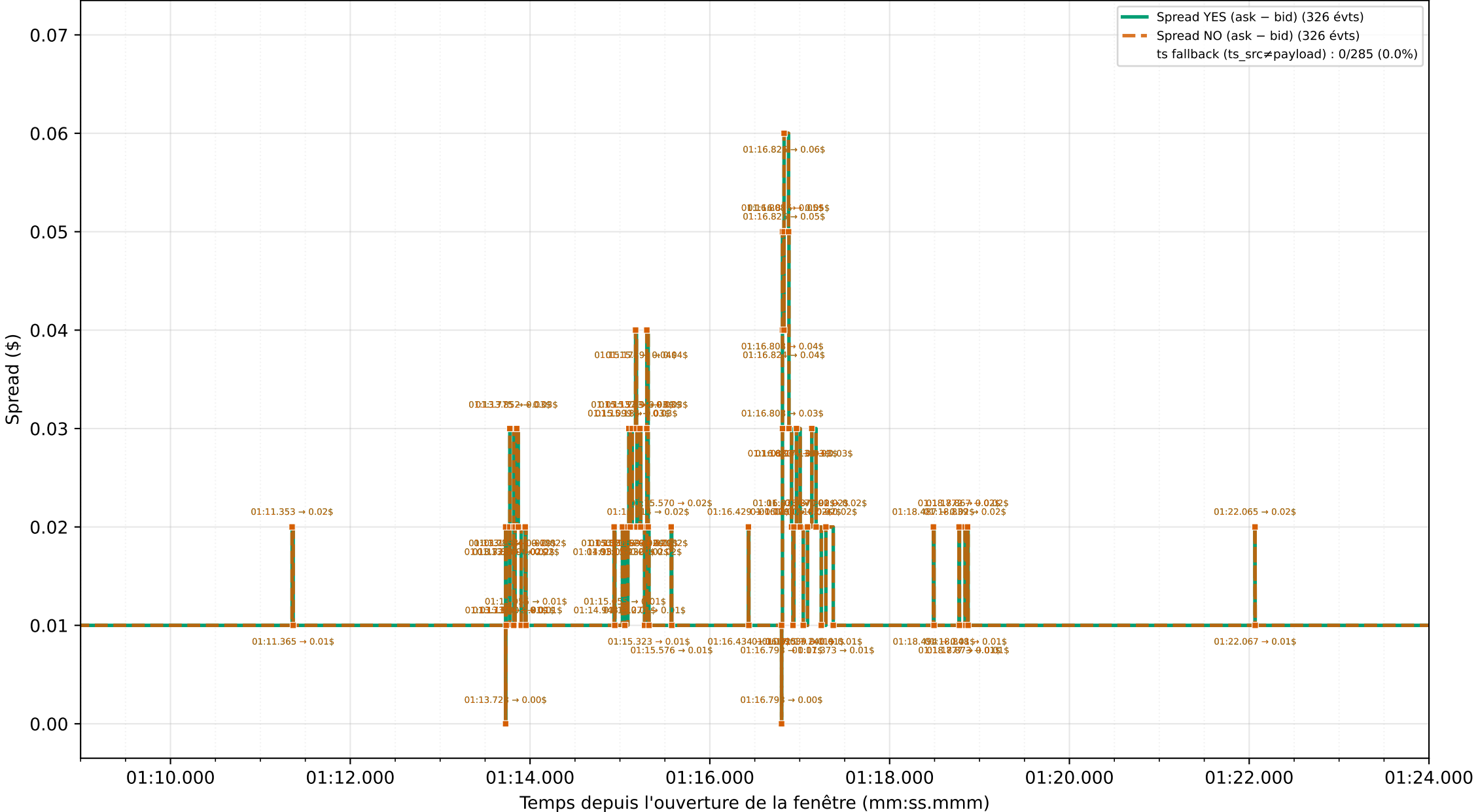
Graphique 5 : Spreads YES et NO absolus (événementiels) — zoom 15 s [01:09.000 → 01:24.000]
