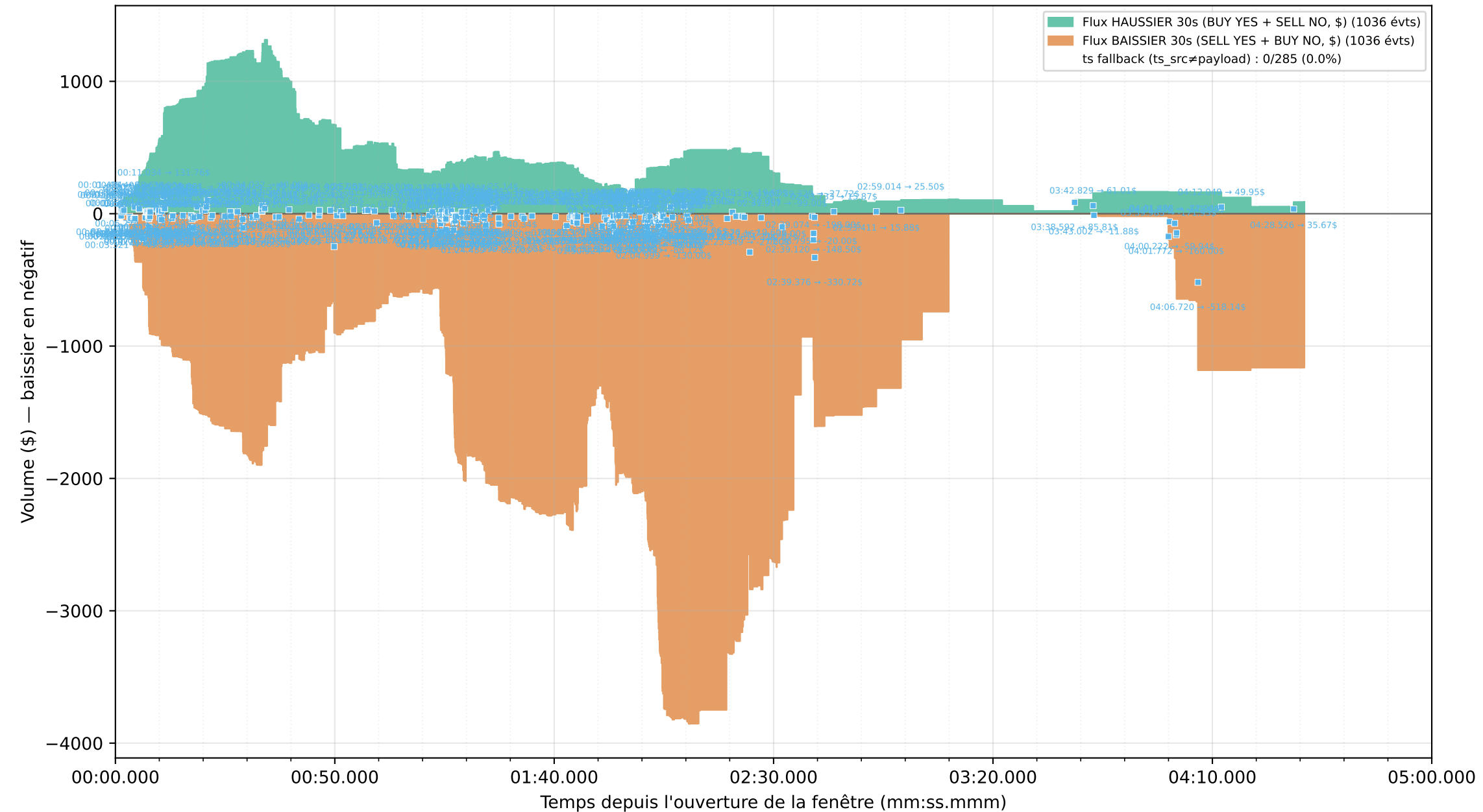
Graphique 3 : Flux directionnel normalisé YES/NO (1036 trades) — vue 300 s
