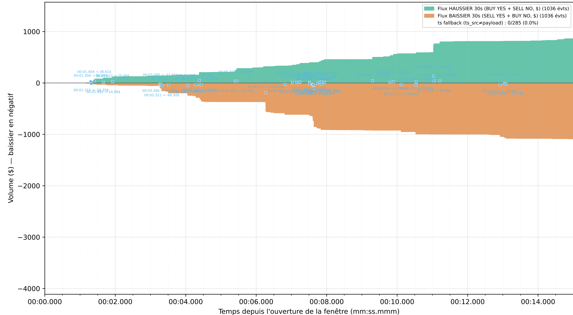
Graphique 3 : Flux directionnel normalisé YES/NO (1036 trades) — zoom 15 s [00:00.000 → 00:15.000]
