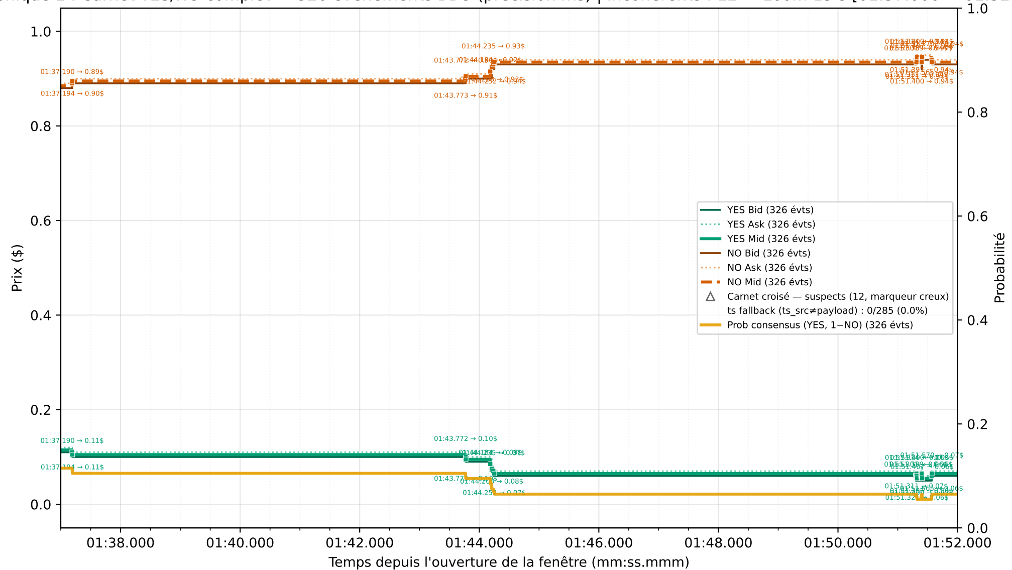
Polymarket BTC 5min | Bitcoin Up or Down - August 18, 9:15AM-9:20AM ET | Résultat : ▼ DOWN Graphique 1 : Carnet YES/NO complet — 326 événements BBO (précision ms) | incohérents : 12 — zoom 15 s [01:37.000 → 01:52.000]
