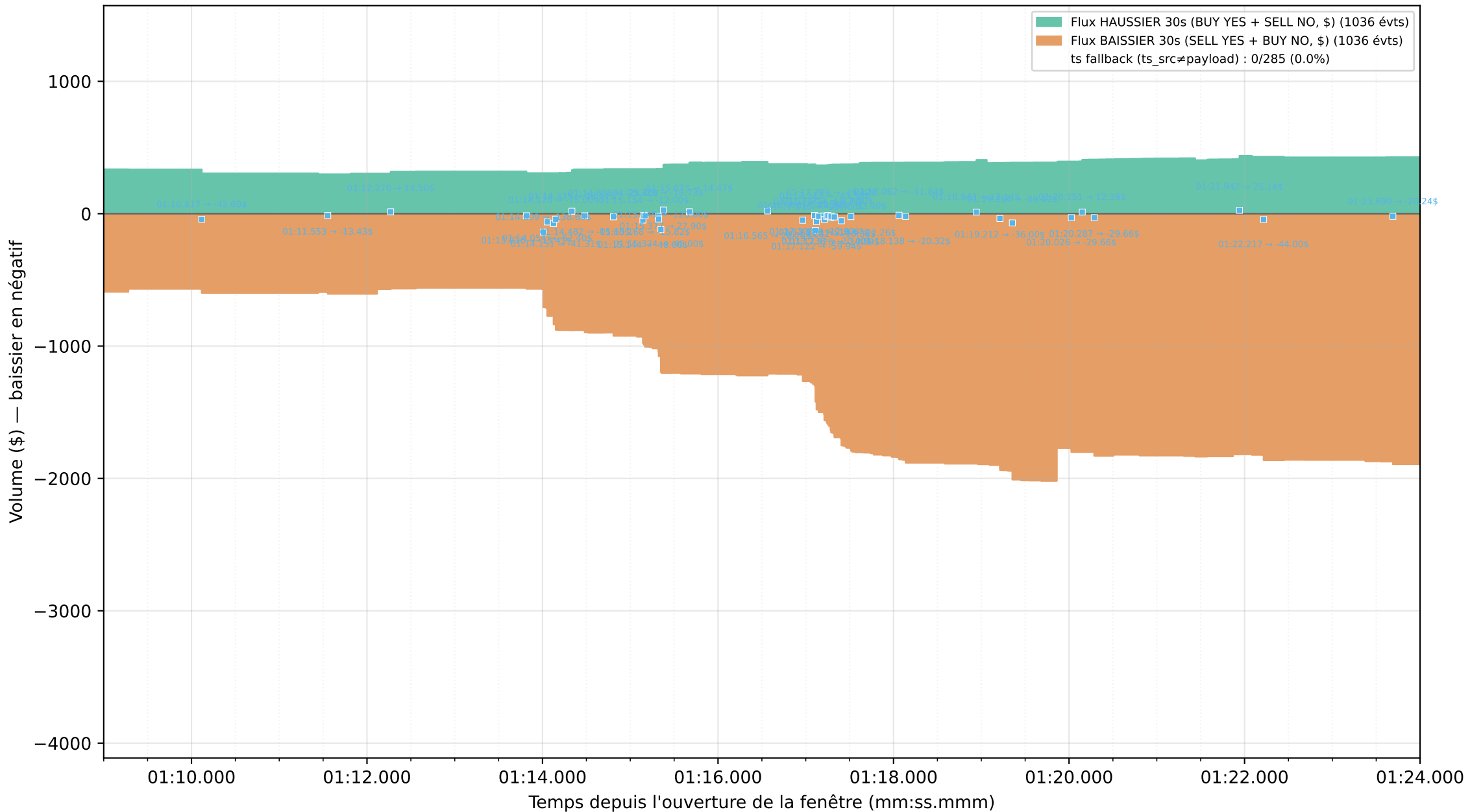
Graphique 3 : Flux directionnel normalisé YES/NO (1036 trades) — zoom 15 s [01:09.000 → 01:24.000]
