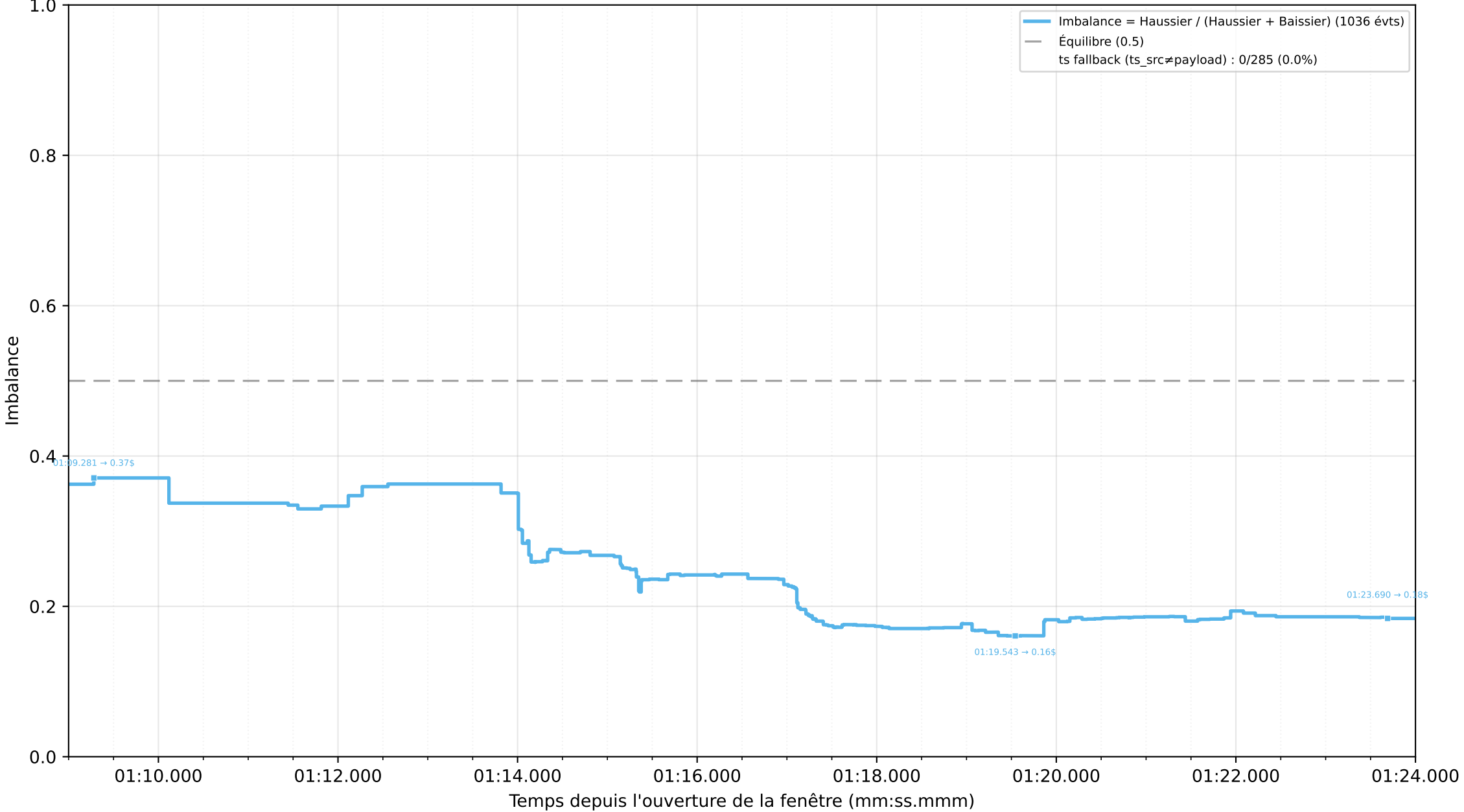
Graphique 4 : Imbalance directionnelle (YES/NO normalisés) — zoom 15 s [01:09.000 → 01:24.000]
