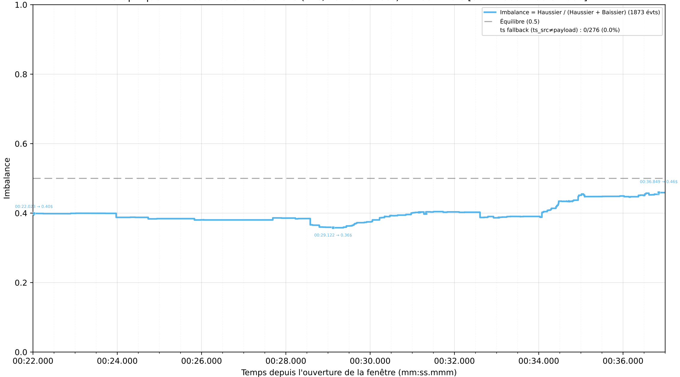
Graphique 4 : Imbalance directionnelle (YES/NO normalisés) — zoom 15 s [00:22.000 → 00:37.000]
