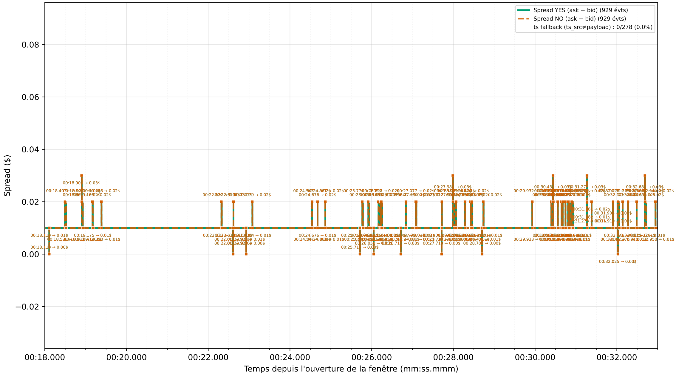
Graphique 5 : Spreads YES et NO absolus (événementiels) — zoom 15 s [00:18.000 → 00:33.000]
