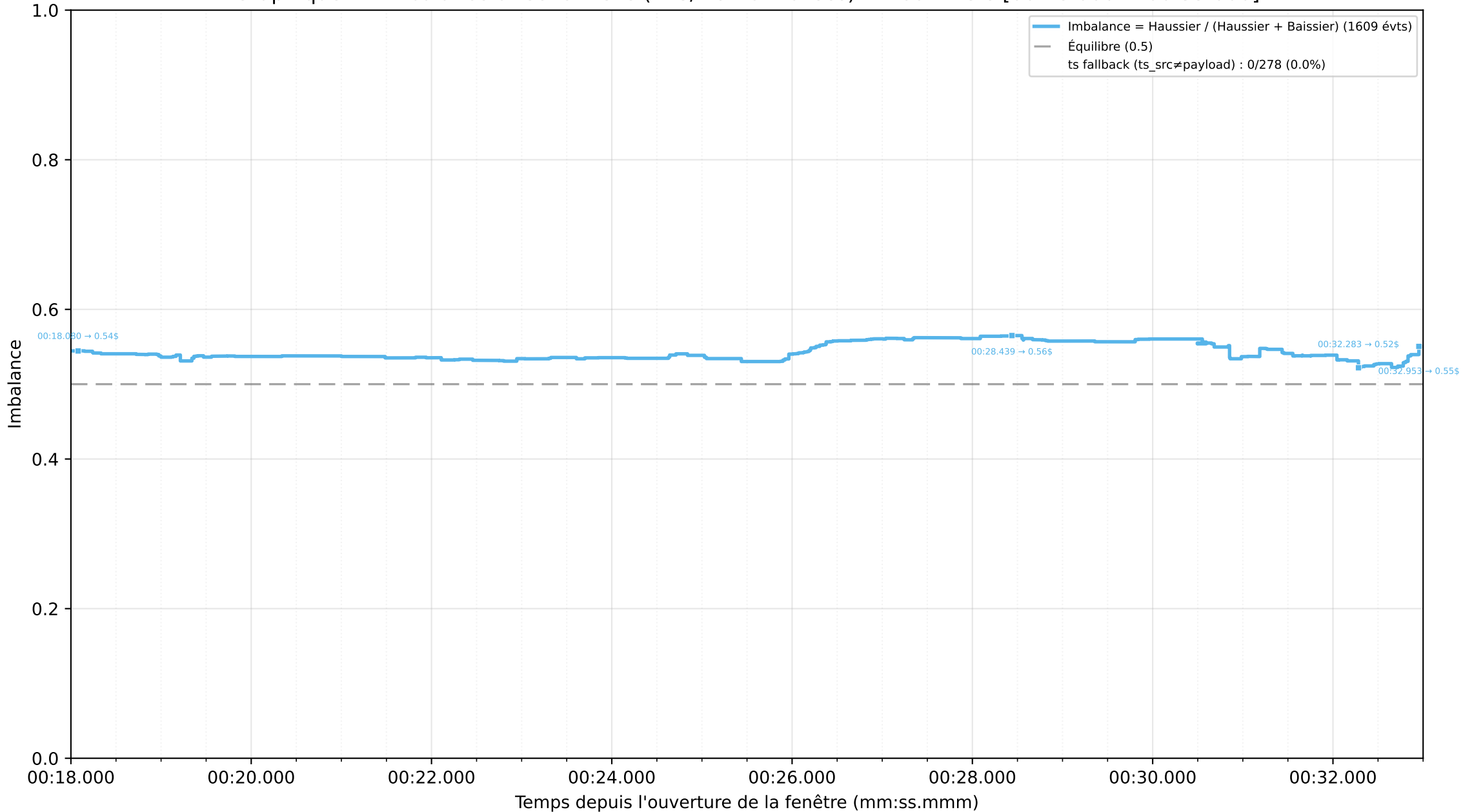
Graphique 4 : Imbalance directionnelle (YES/NO normalisés) — zoom 15 s [00:18.000 → 00:33.000]
