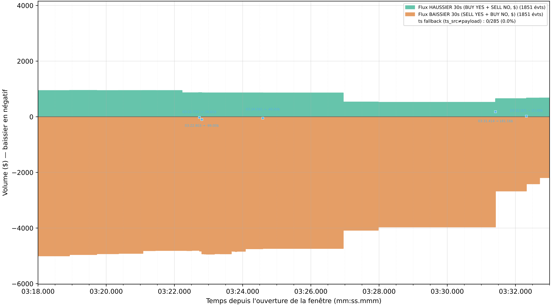
Graphique 3 : Flux directionnel normalisé YES/NO (1851 trades) — zoom 15 s [03:18.000 → 03:33.000]
