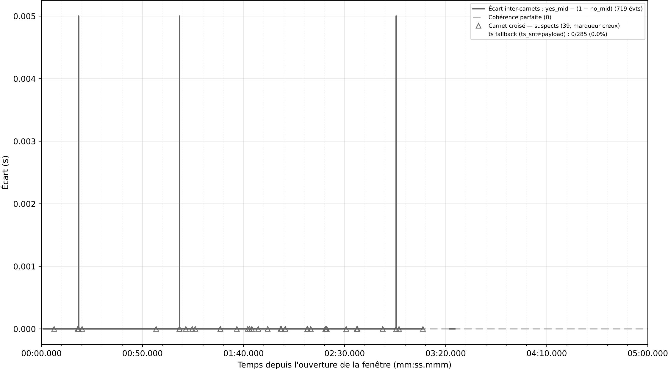
Graphique 6 : Écart inter-carnets YES vs NO (incohérents : 39) — vue 300 s
