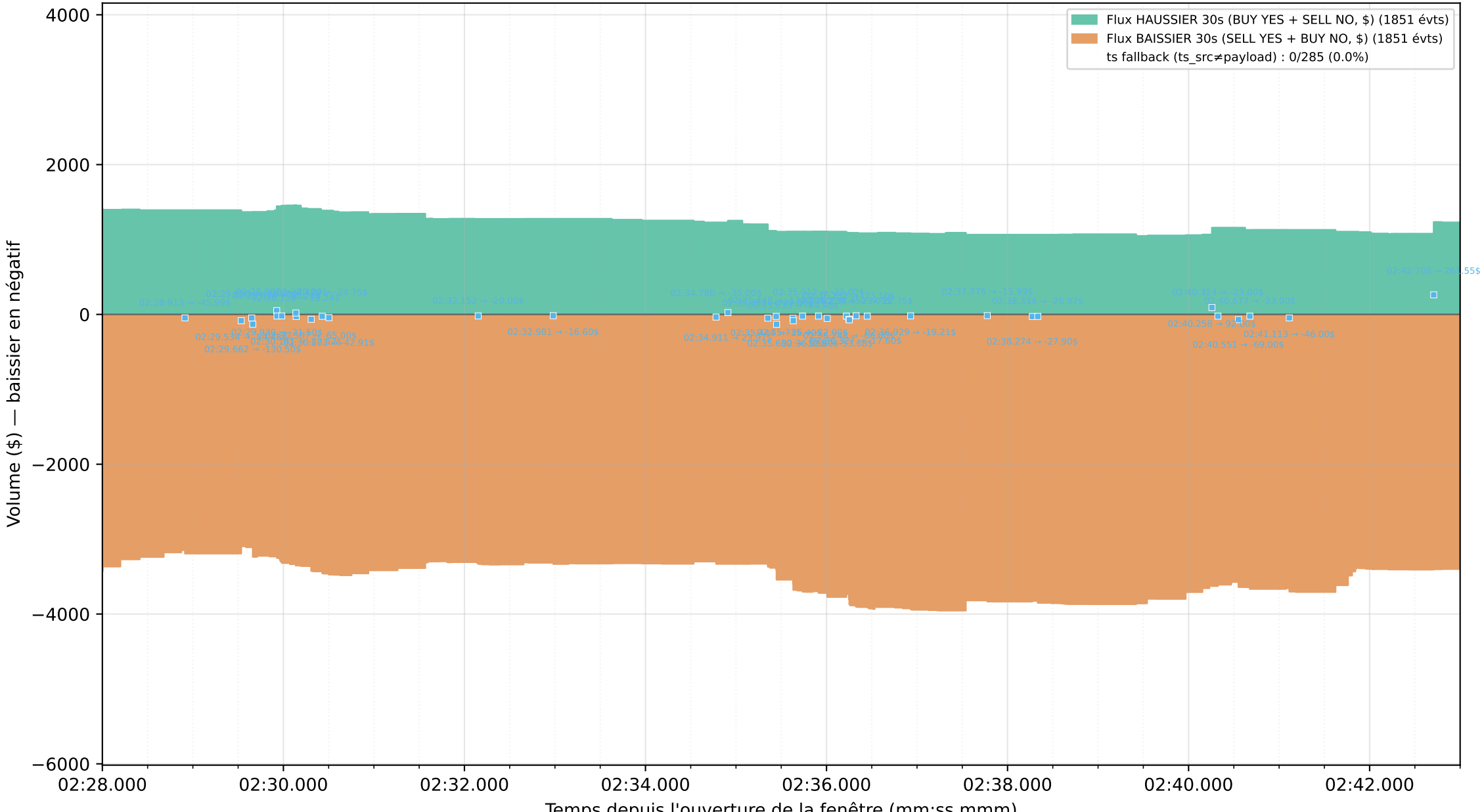
Graphique 3 : Flux directionnel normalisé YES/NO (1851 trades) — zoom 15 s [02:28.000 → 02:43.000]
