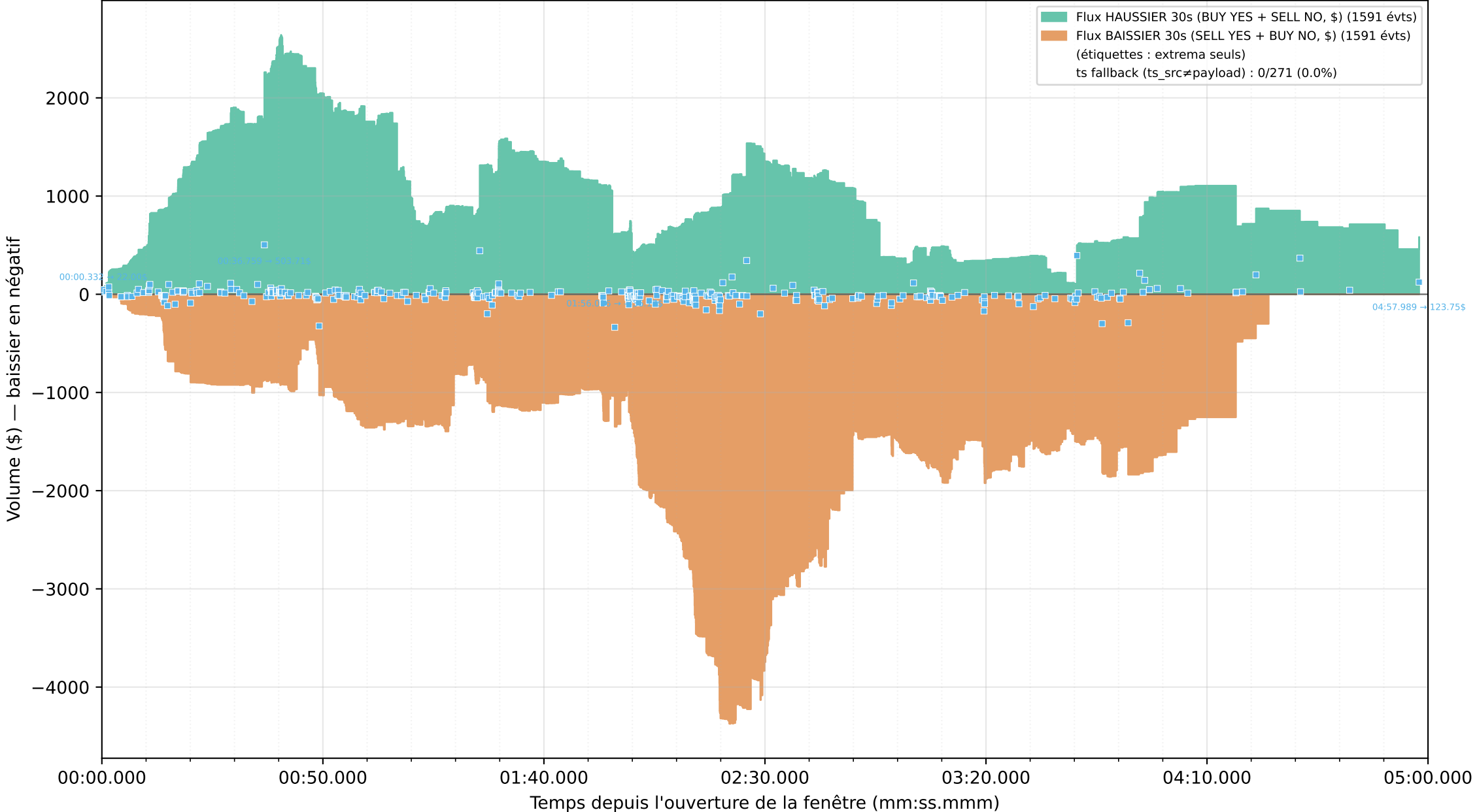
Graphique 3 : Flux directionnel normalisé YES/NO (1591 trades) — vue 300 s
