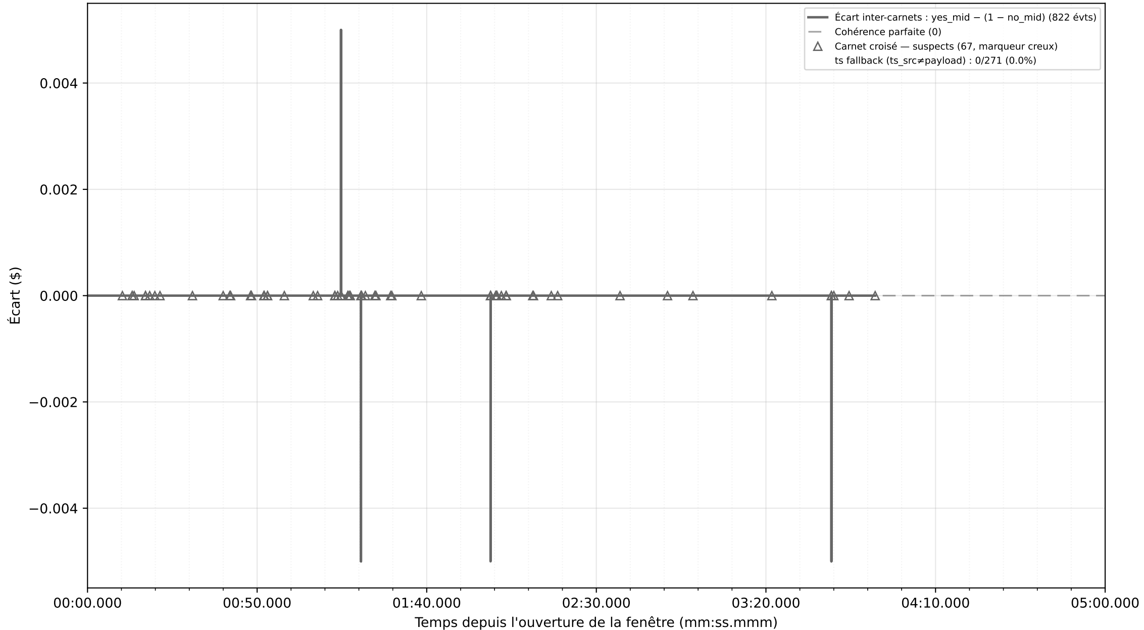
Graphique 6 : Écart inter-carnets YES vs NO (incohérents : 67) — vue 300 s
