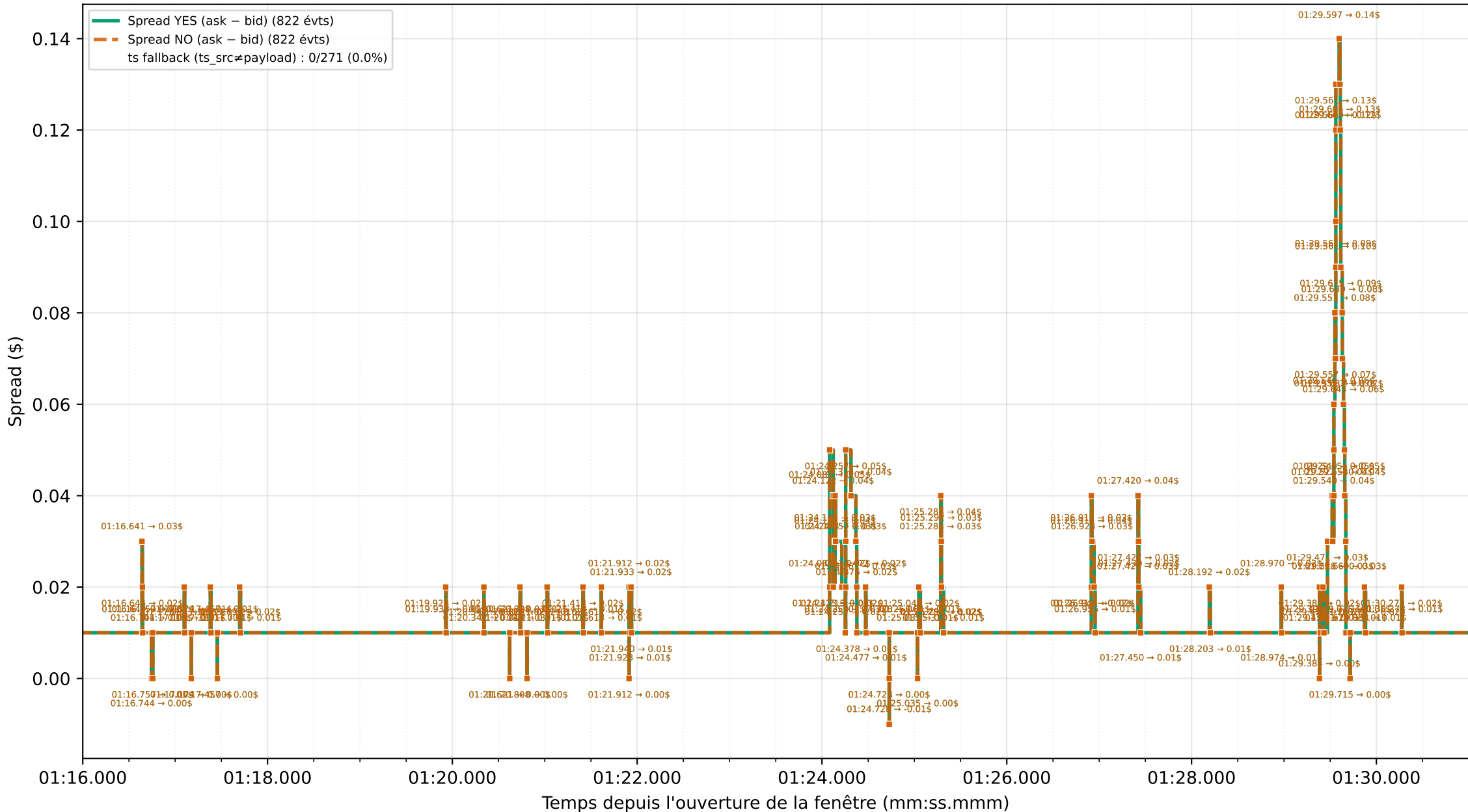
Graphique 5 : Spreads YES et NO absolus (événementiels) — zoom 15 s [01:16.000 → 01:31.000]
