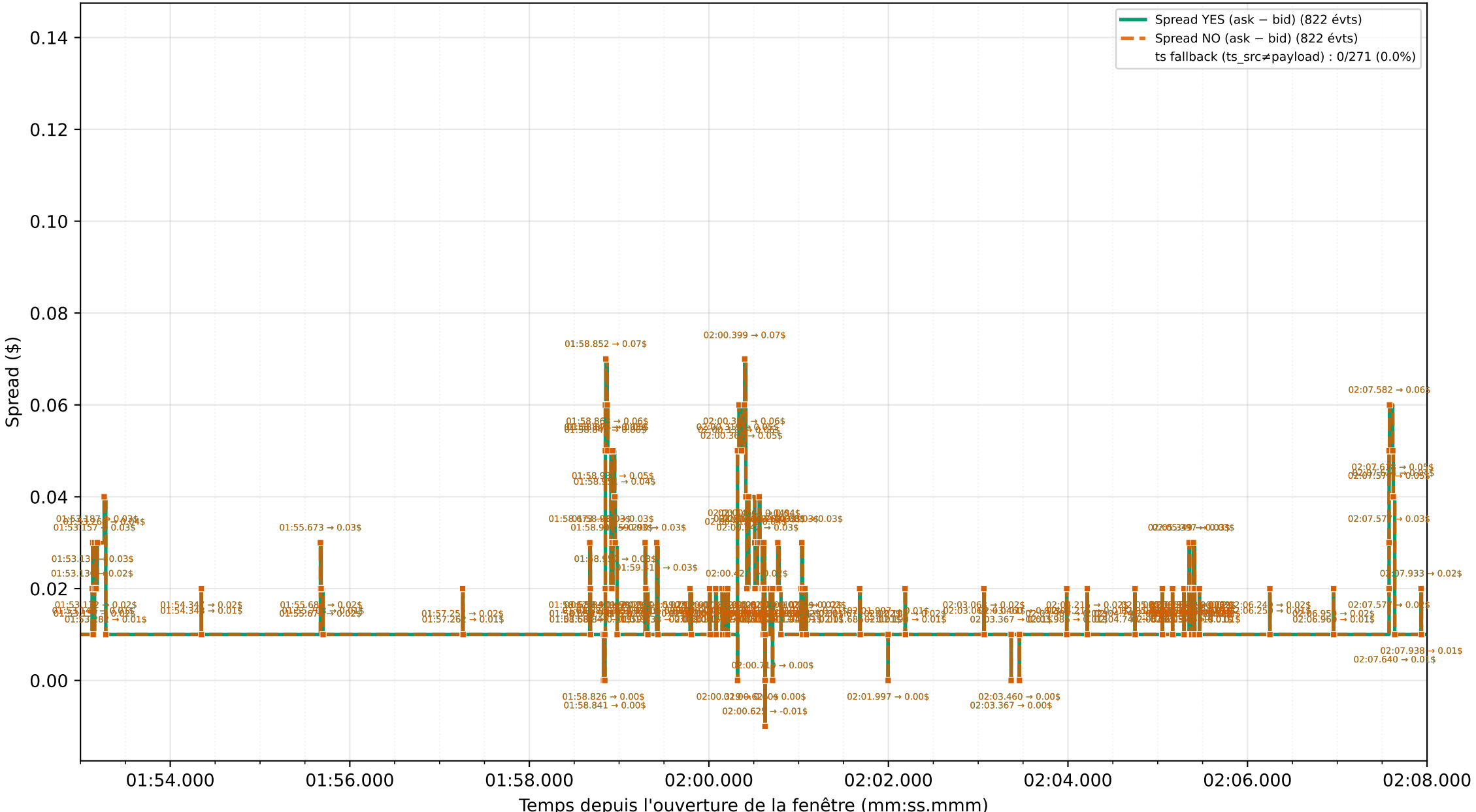
Graphique 5 : Spreads YES et NO absolus (événementiels) — zoom 15 s [01:53.000 → 02:08.000]
