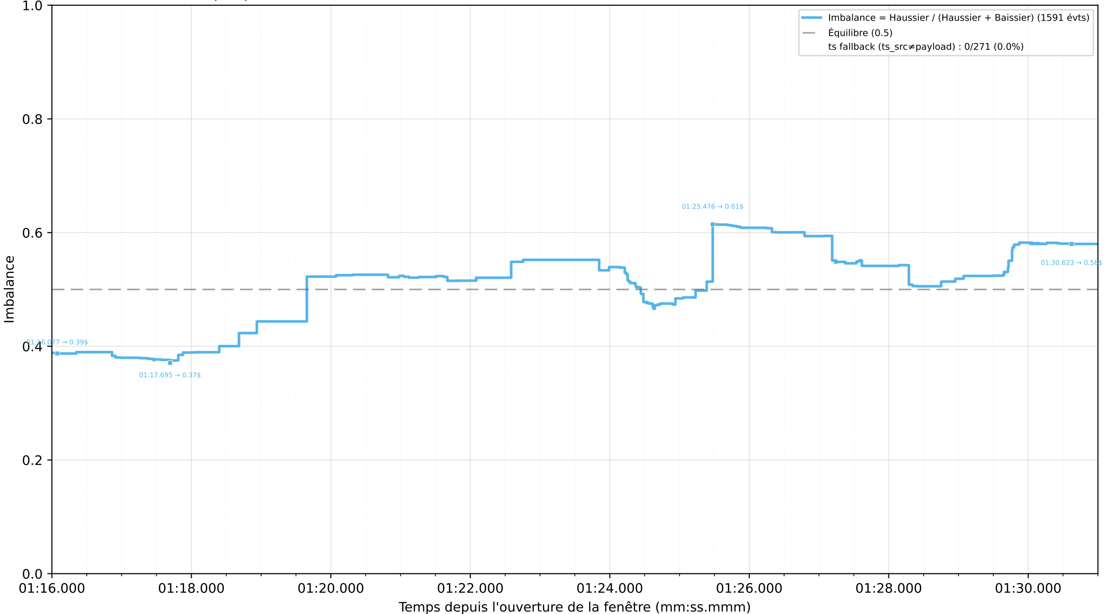
Graphique 4 : Imbalance directionnelle (YES/NO normalisés) — zoom 15 s [01:16.000 → 01:31.000]
