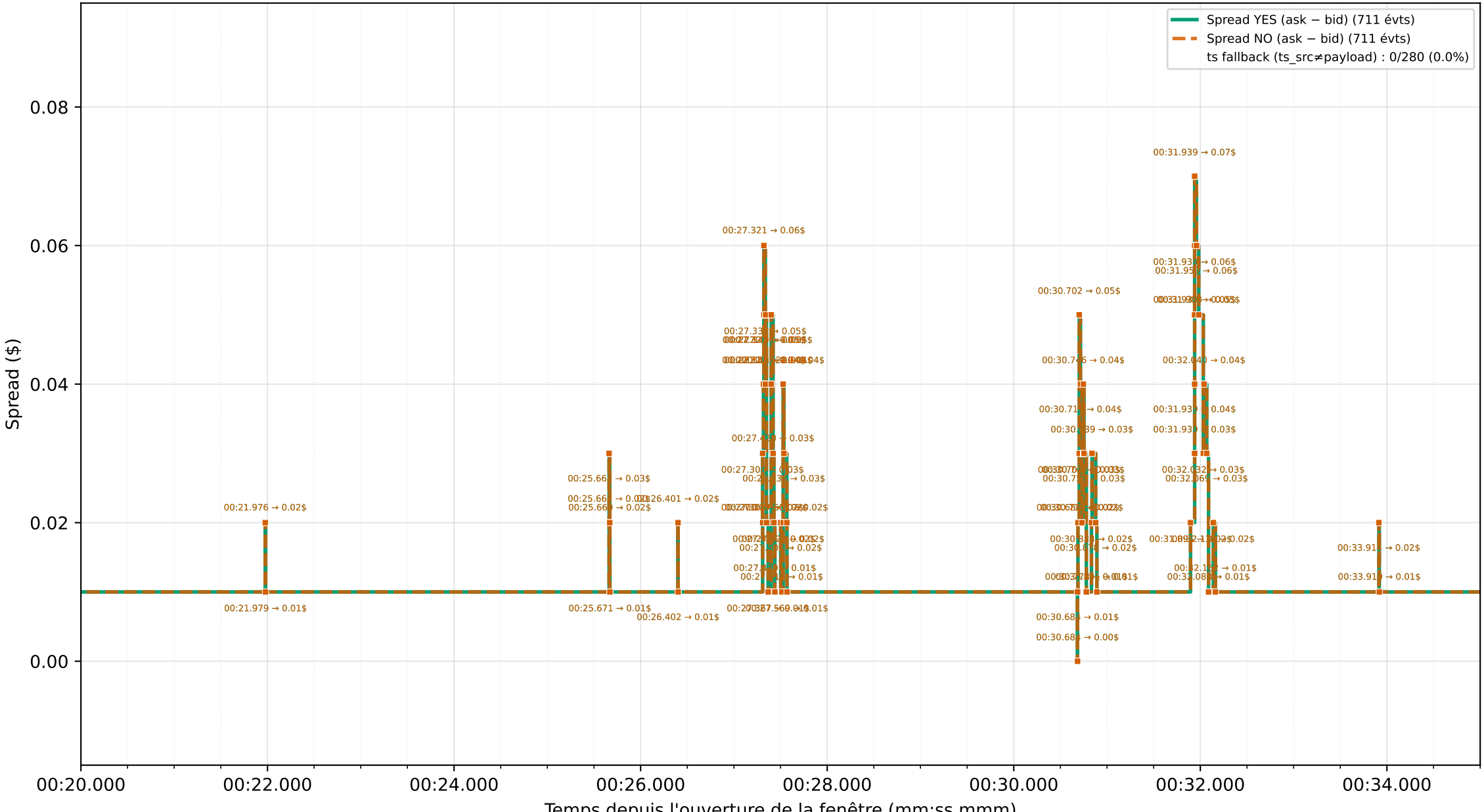
Graphique 5 : Spreads YES et NO absolus (événementiels) — zoom 15 s [00:20.000 → 00:35.000]
