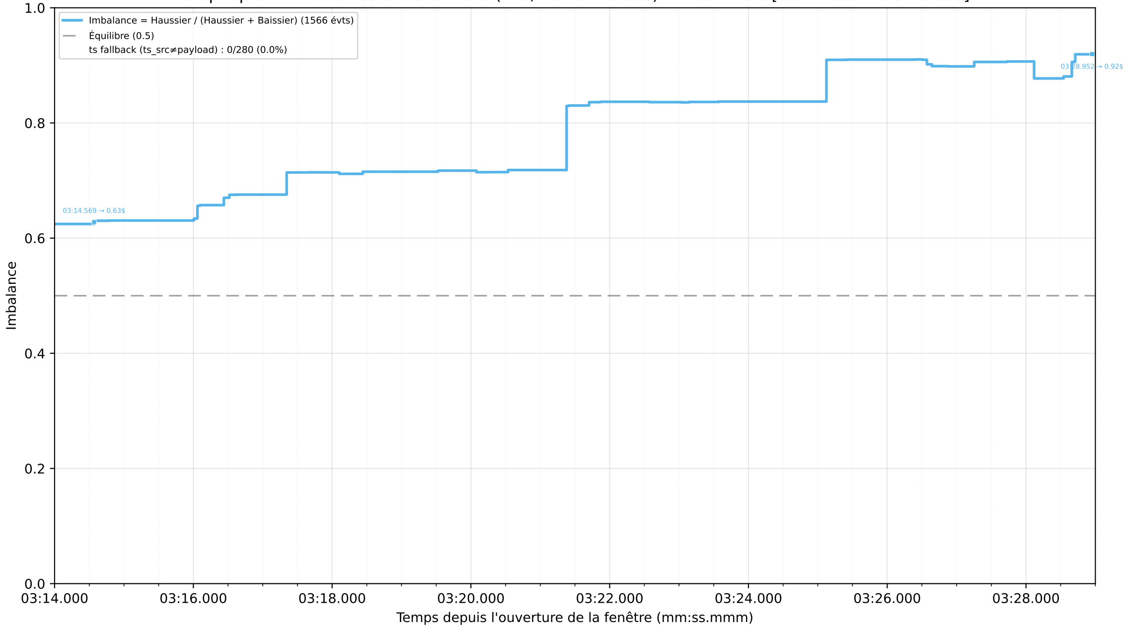
Graphique 4 : Imbalance directionnelle (YES/NO normalisés) — zoom 15 s [03:14.000 → 03:29.000]
