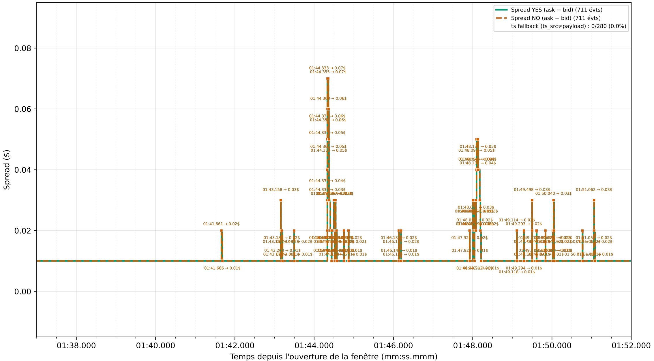
Graphique 5 : Spreads YES et NO absolus (événementiels) — zoom 15 s [01:37.000 → 01:52.000]
