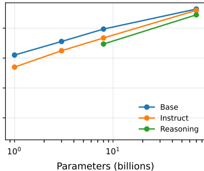
Llama3.X
