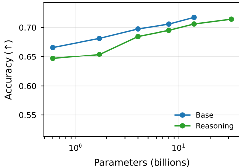
Qwen3
