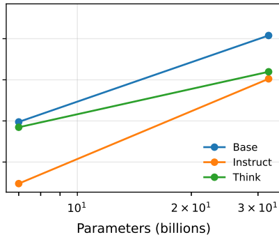
Olmo3.X
