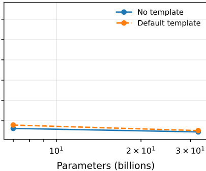
Olmo3.X
