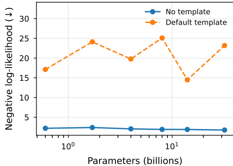
Qwen3
