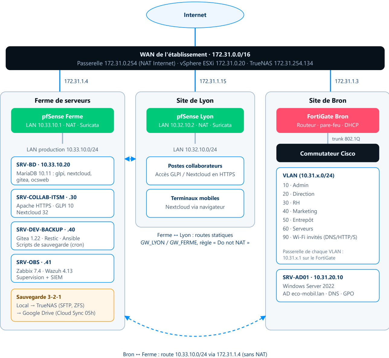
Schéma logique de l'infrastructure EcoMobil (adresses de production et de gestion).
