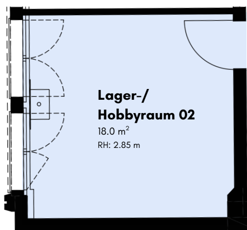
Massstab 1:75 RH = Raumhöhe
