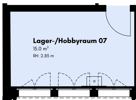
Massstab 1:75 RH = Raumhöhe
