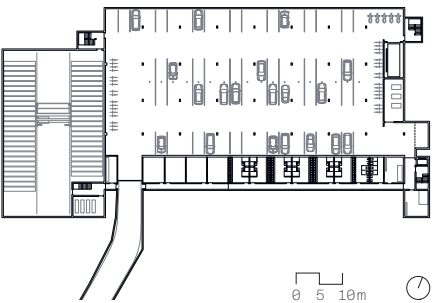
Untergeschoss
