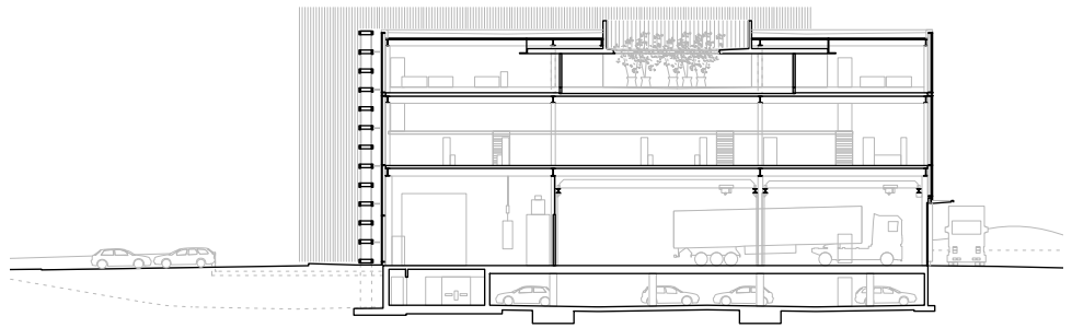
Schnitt 1:600
