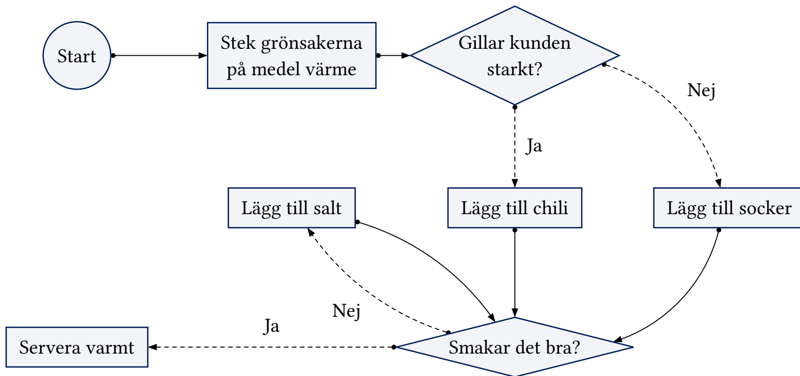
Figur 3: Flödesschema för matlagningsalgoritmen
