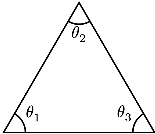
Figur 1: En liksidig triangel
