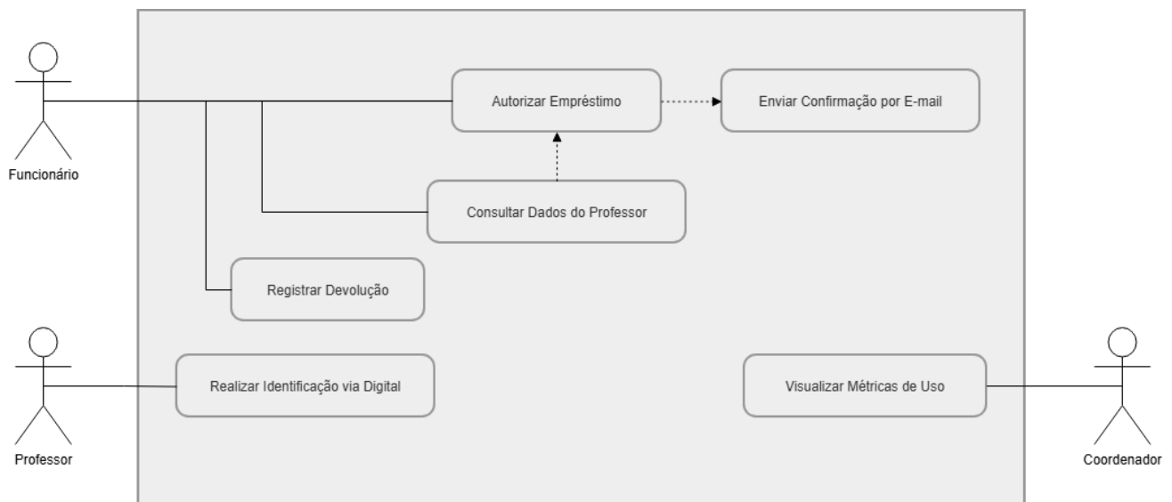
Figura 1 — Diagrama de Caso de Uso: Sistema de Empréstimo de Projetores CCT/Unifor
