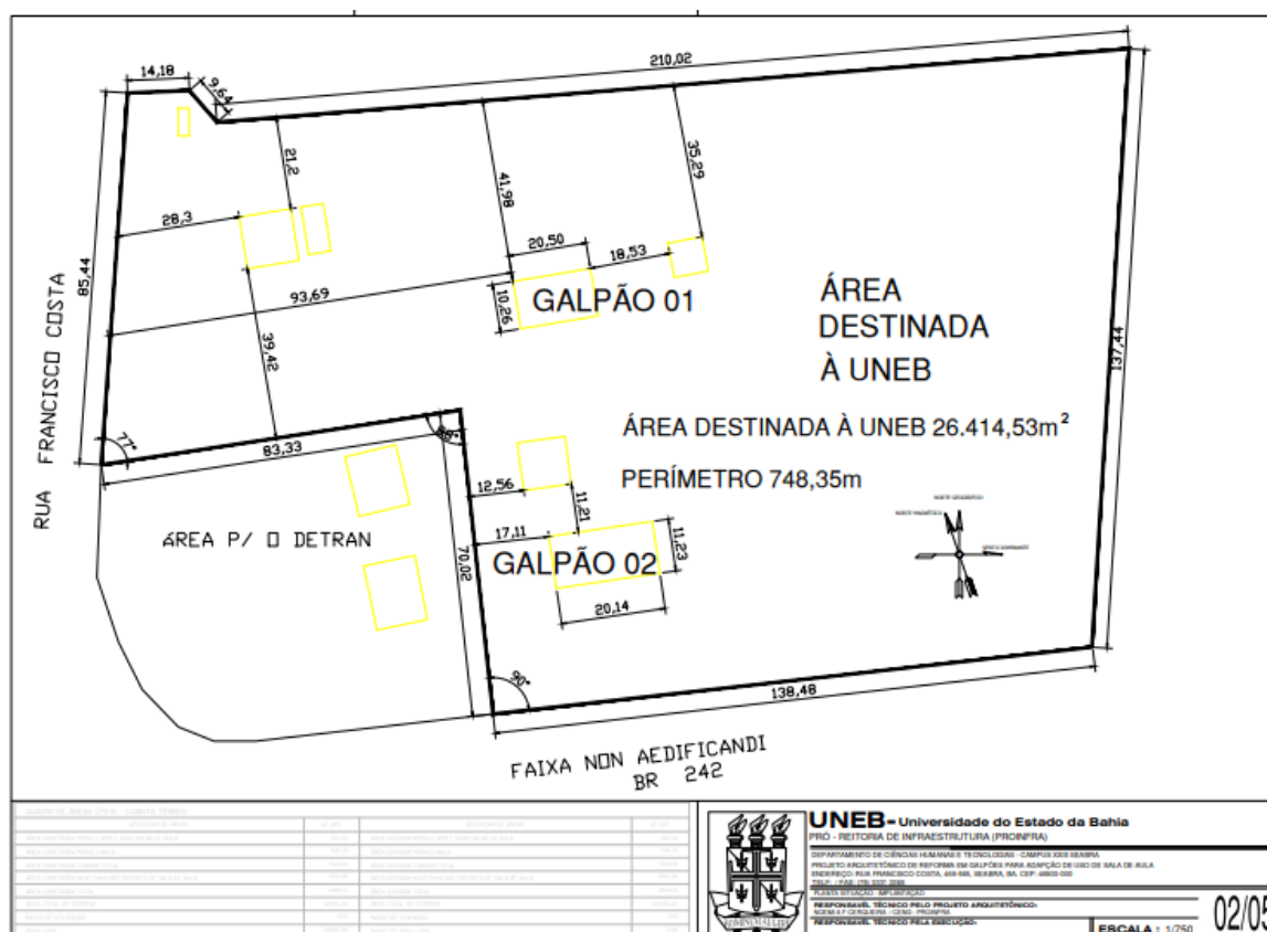
Figura 01 – Planta da nova sede
