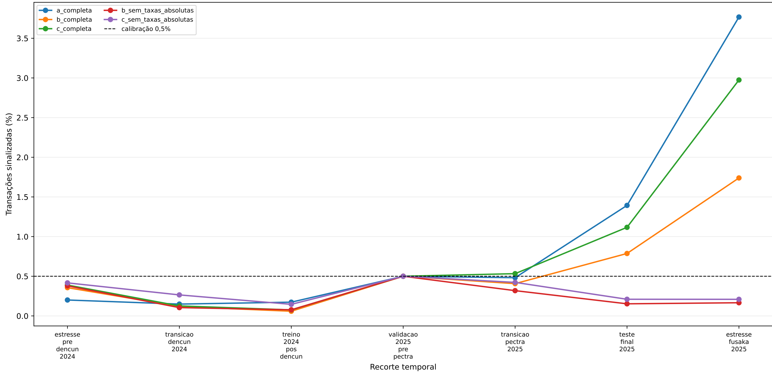
Isolation Forest: taxa de anomalias pelo limiar Q99,5 da validação
