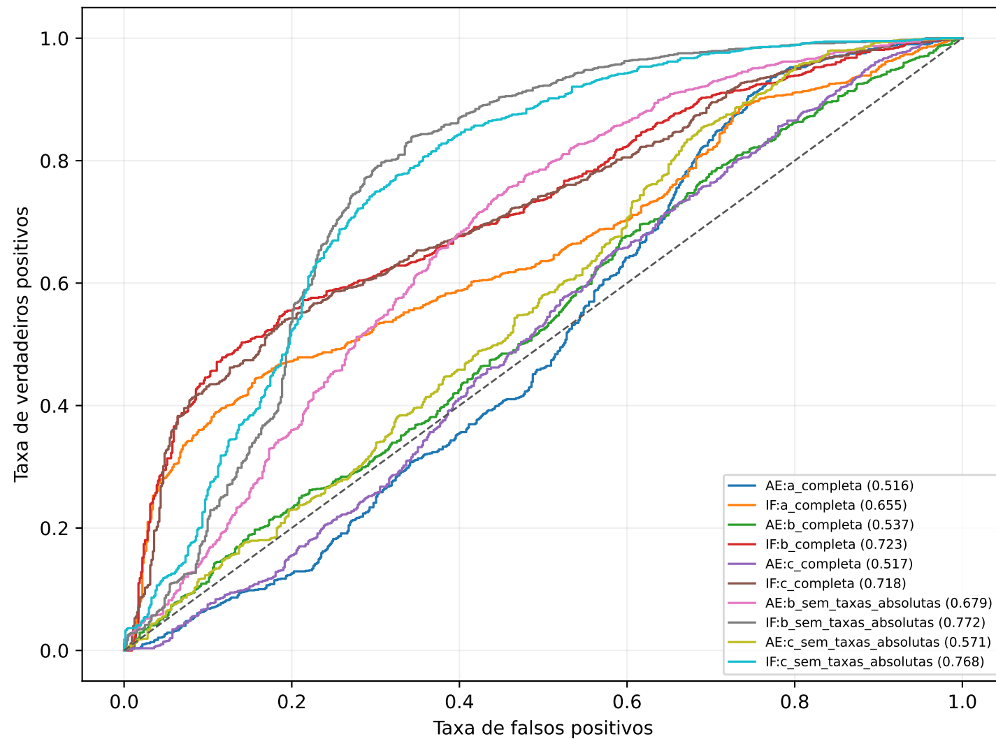
Curvas ROC
