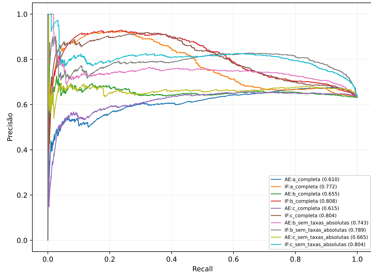
Curvas Precision-Recall
