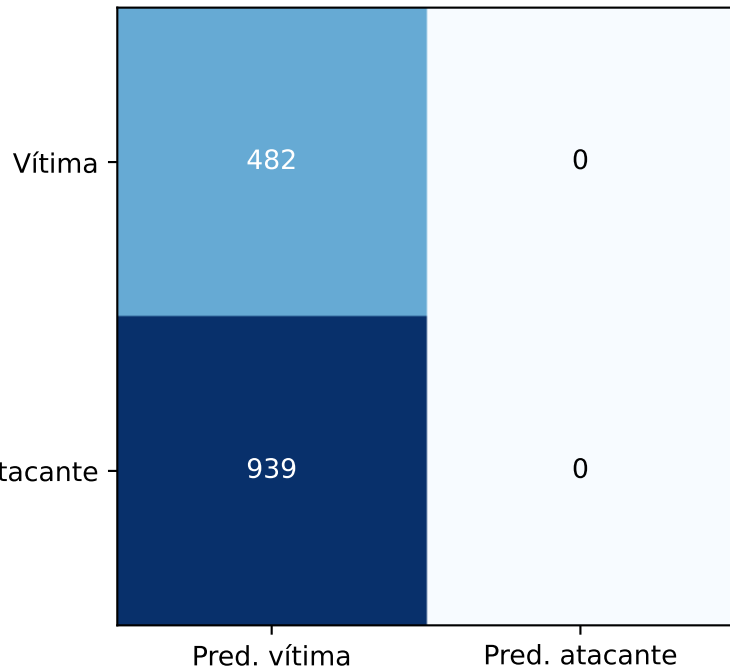
AE:b_sem_texas_absolutas — q990
