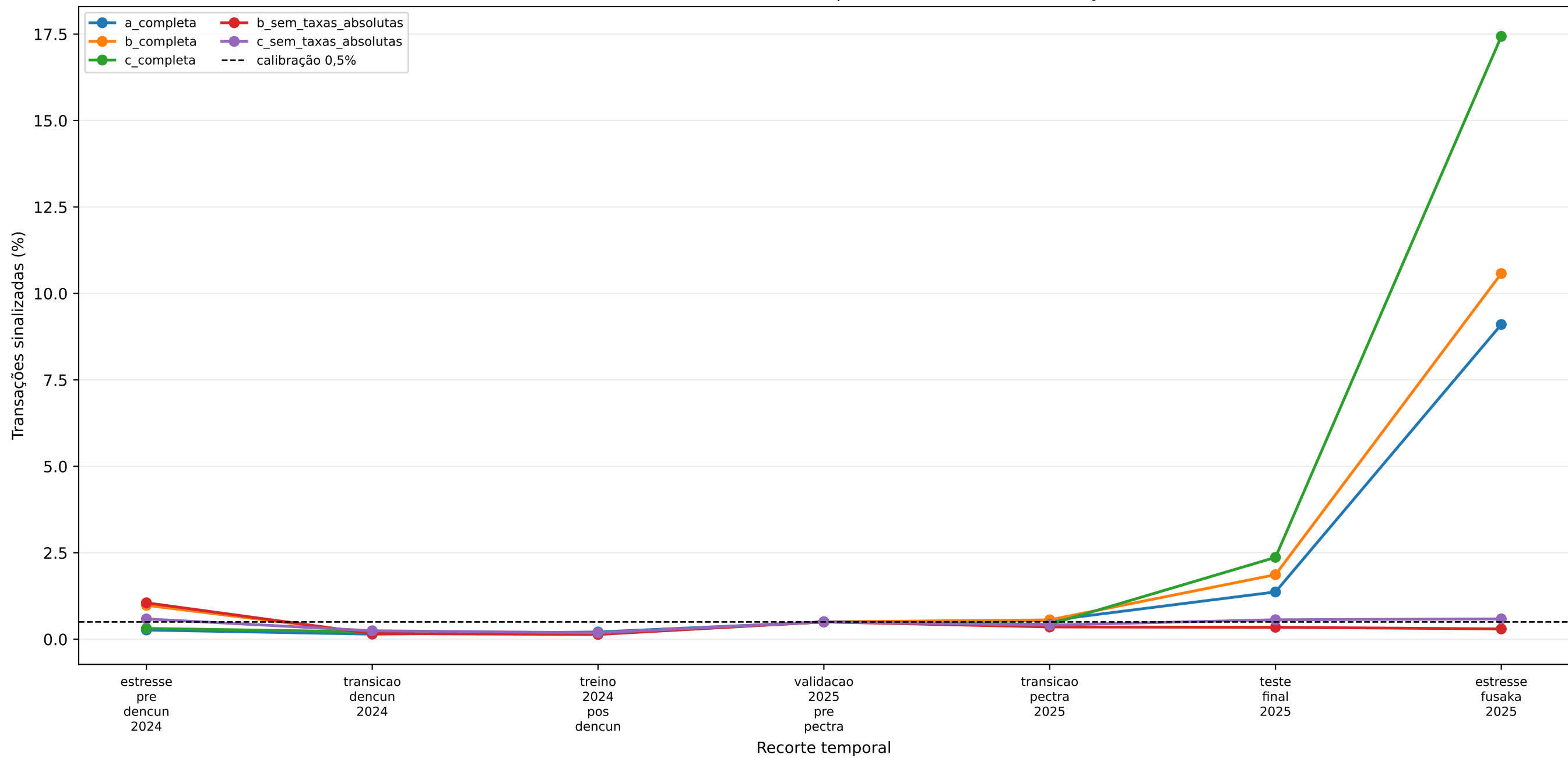
Autoencoder: taxa de anomalias pelo limiar Q99,5 da validação
