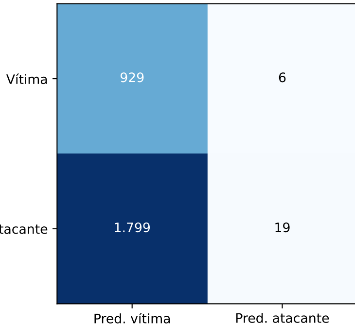
AE:c_sem_texas_absolutas — q990
