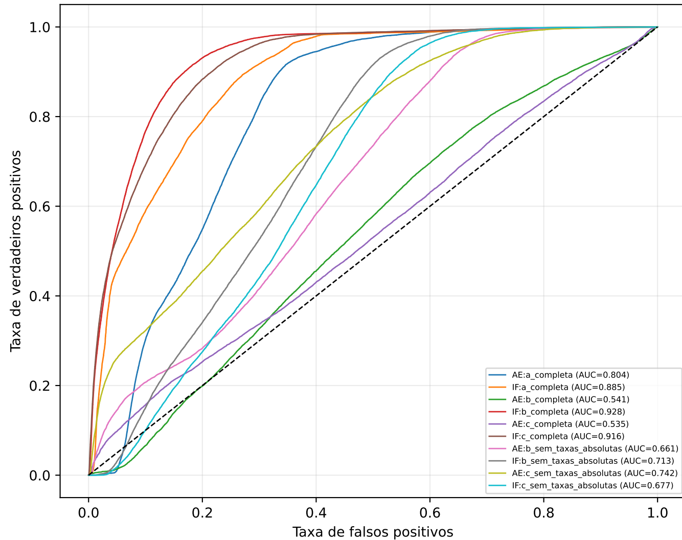
Curvas ROC
