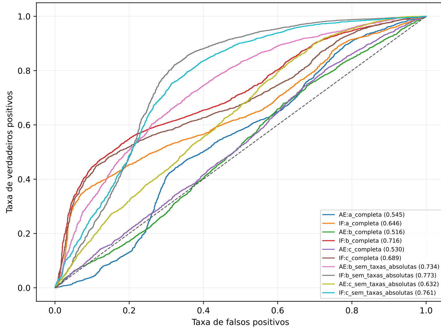
Curvas ROC
