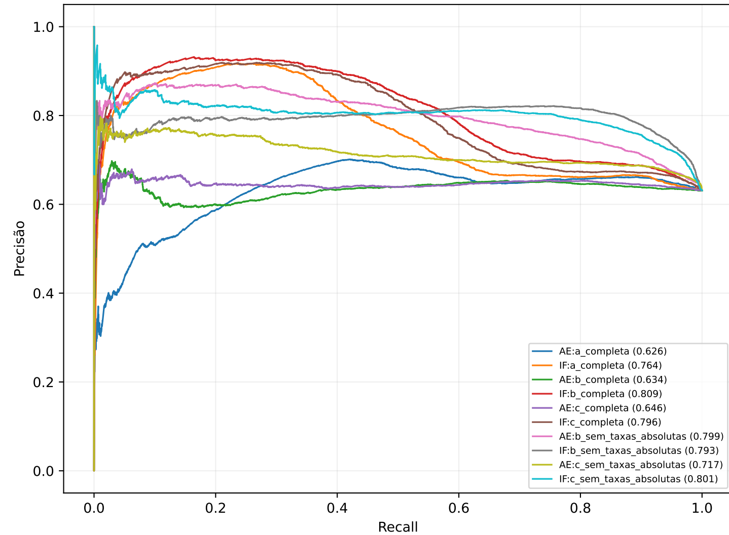
Curvas Precision-Recall
