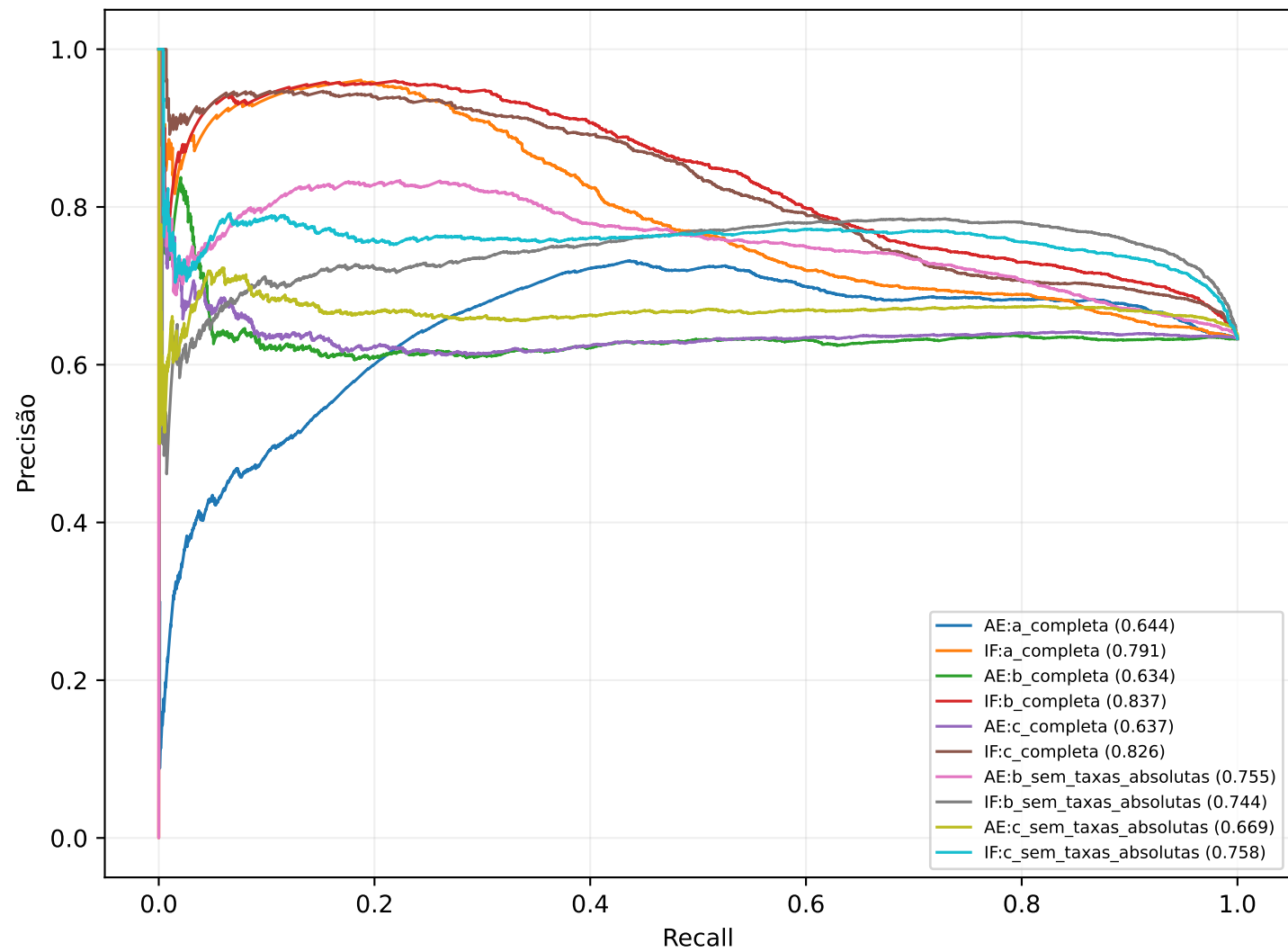
Curvas Precision-Recall
