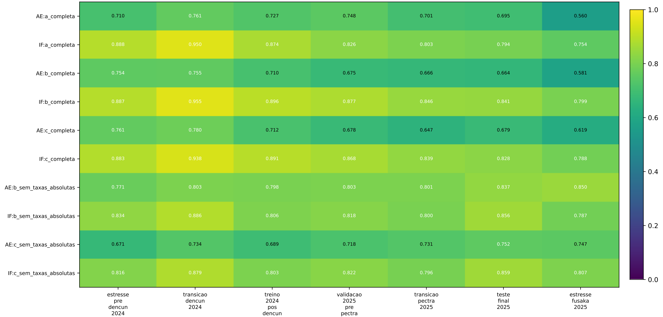
PR-AUC por janela — política strict
