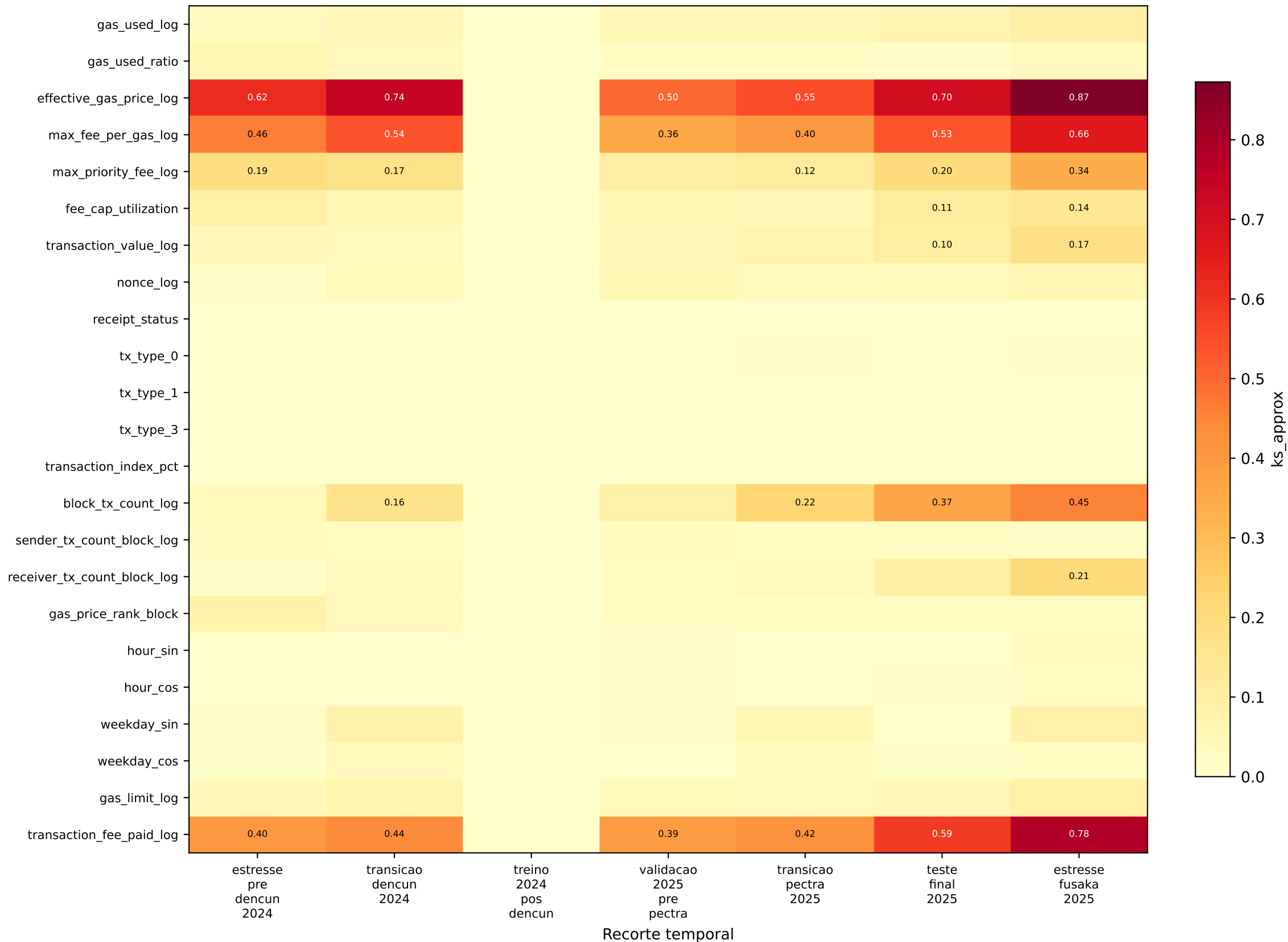
Distância KS aproximada por feature e recorte
