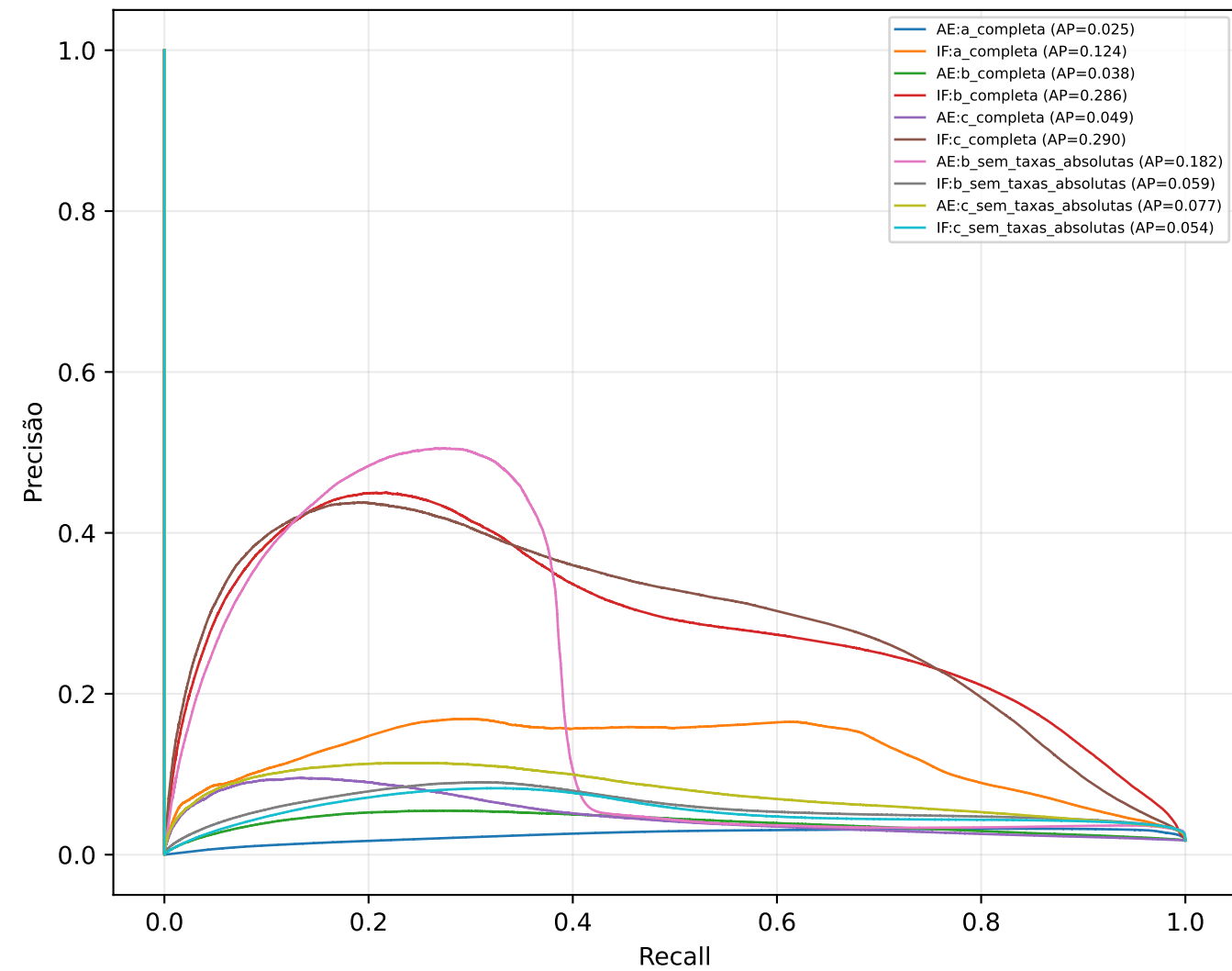
Curvas Precision-Recall
