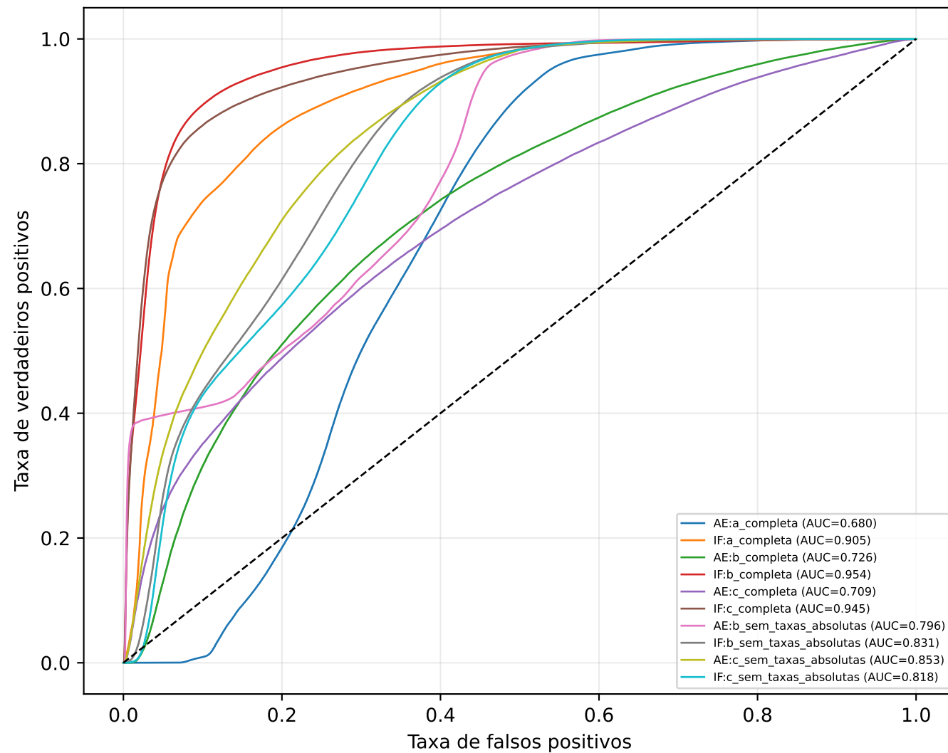
Curvas ROC
