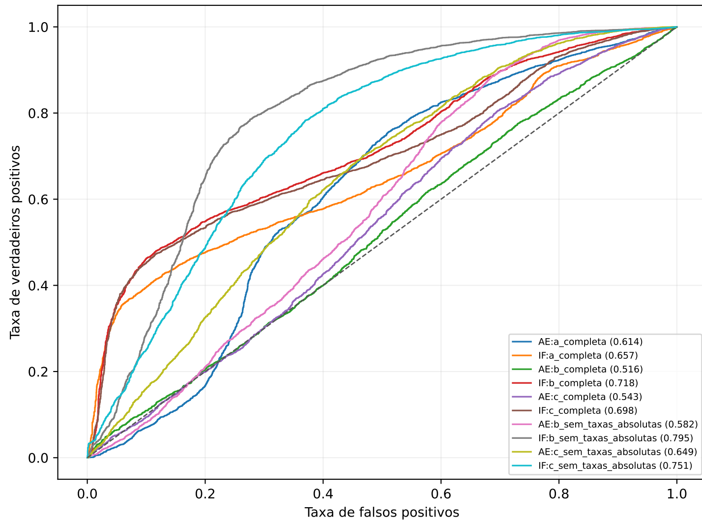
Curvas ROC
