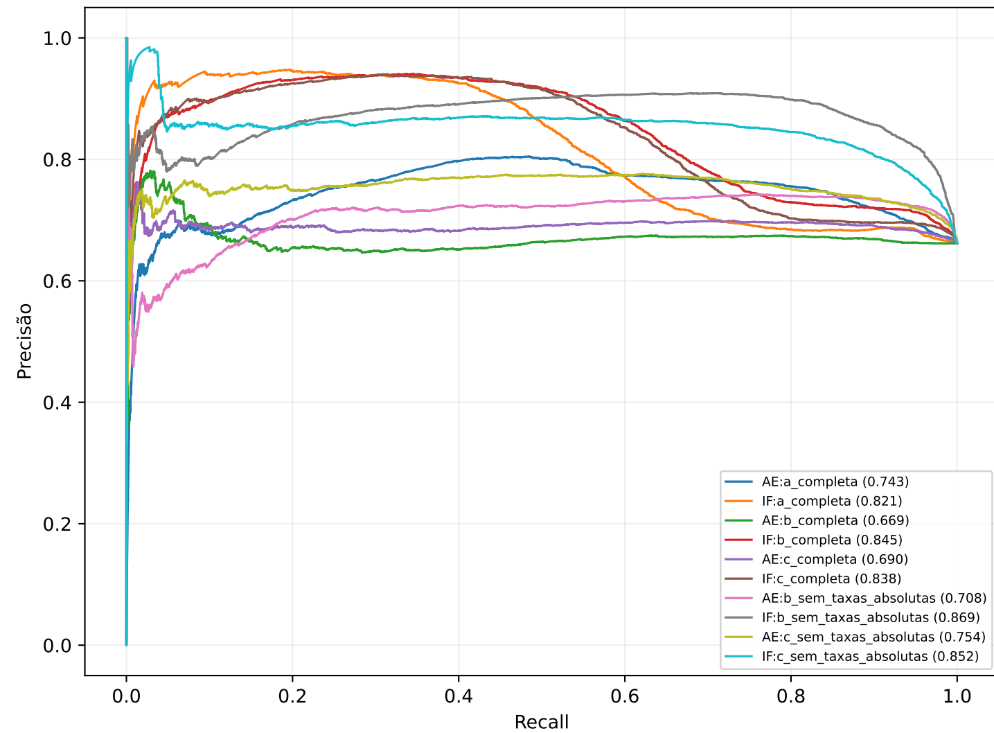
Curvas Precision-Recall
