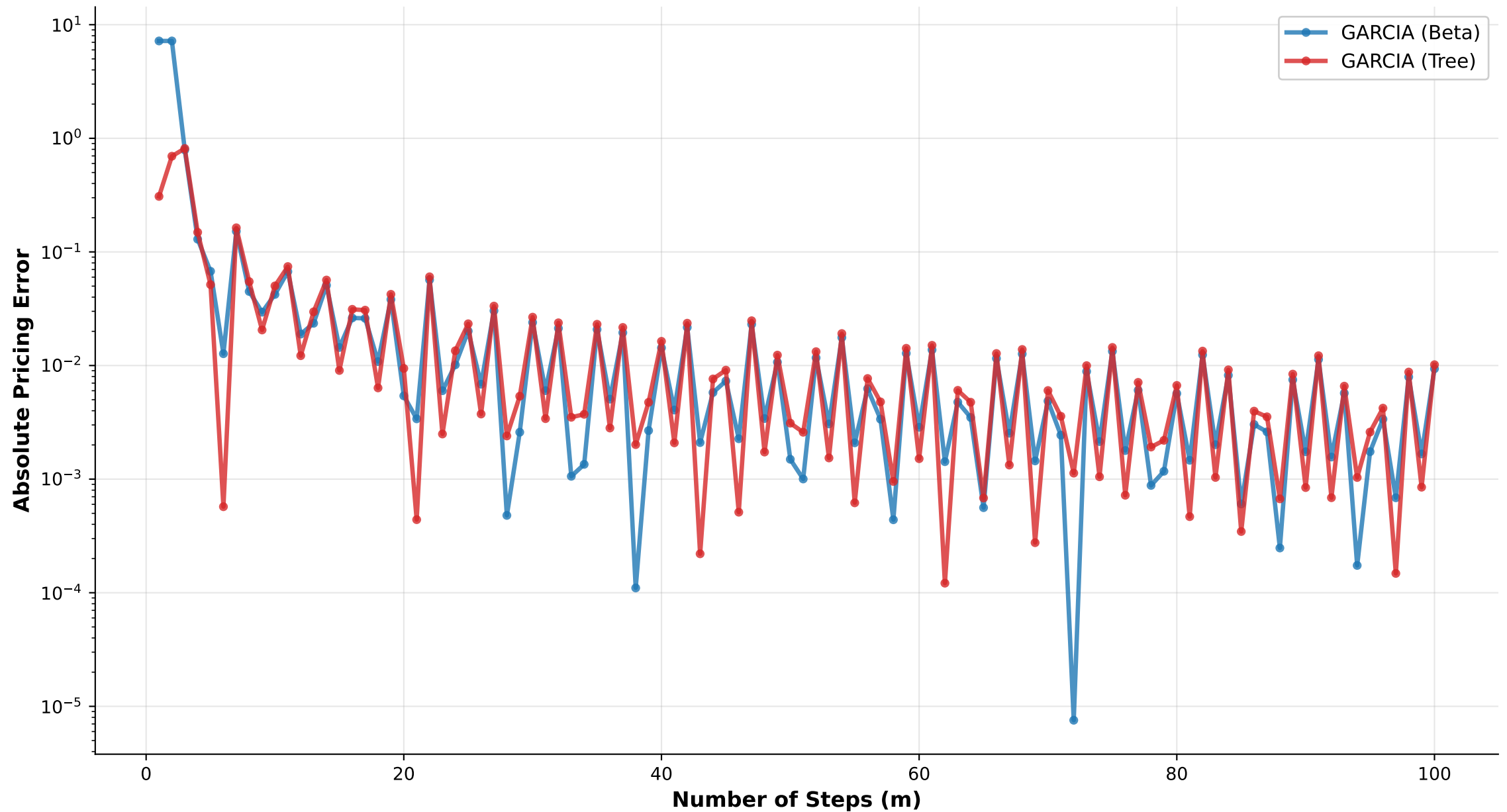
Vanilla Put: Beta-Binomial vs Binomial Tree (Garcia)
