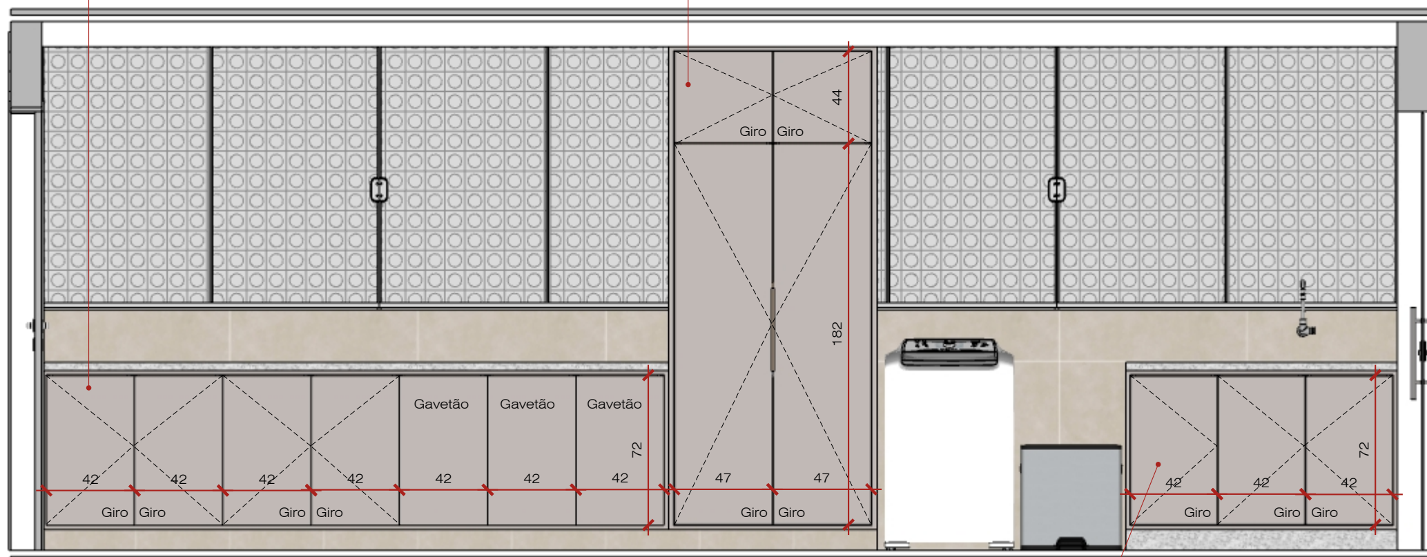
Vista E - Área de Serviço - Marcenaria Externa Esc: 1/25
