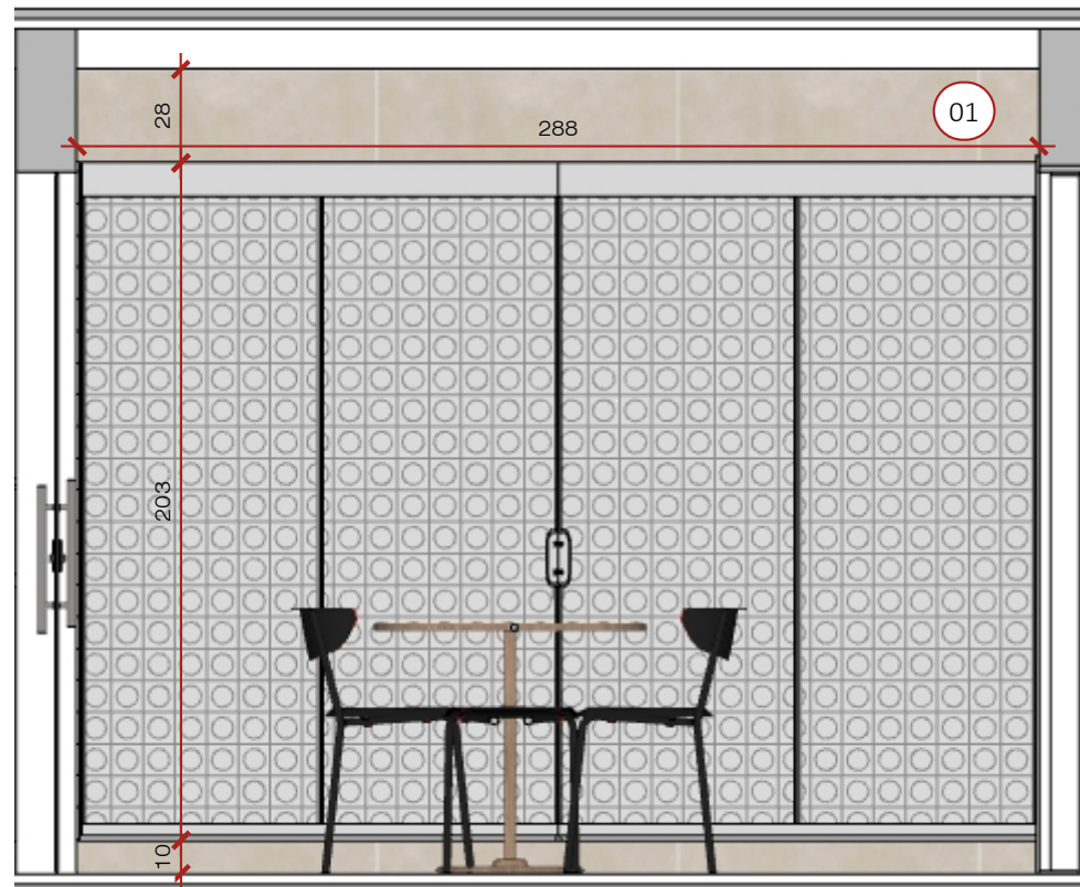
Vista D - Cozinha - Paginação Esc: 1/25
