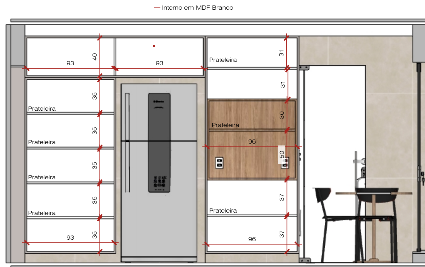
Vista C - Cozinha - Marcenaria Interna Esc: 1/25
