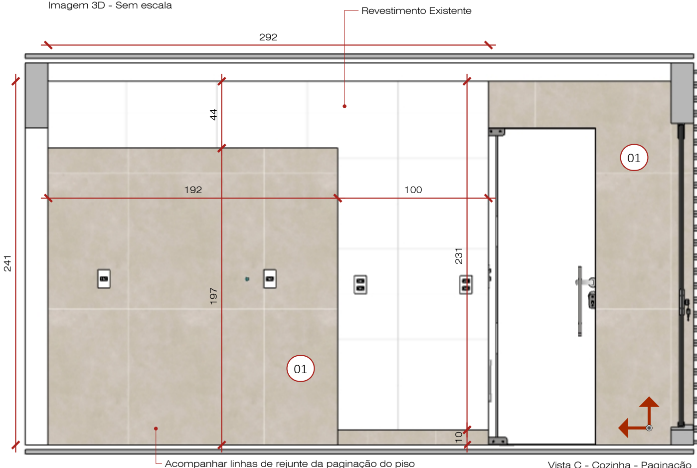
Vista C - Cozinha - Paginação Esc: 1/25
