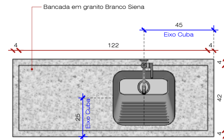
Vista E - Área de Serviço - Marmoraria Esc: 1/15
