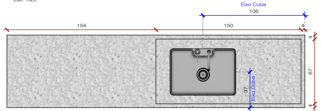
Vista A - Detalhe - Marmoraria Esc: 1/25
