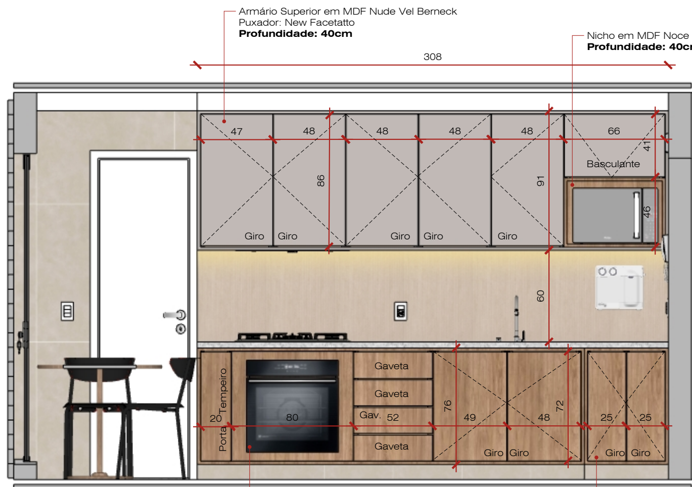
Vista A - Cozinha - Marcenaria Externa Esc: 1/25
