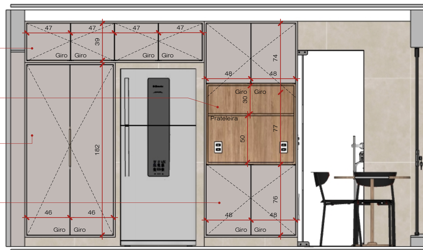
Vista C - Cozinha - Marcenaria Externa Esc: 1/25
