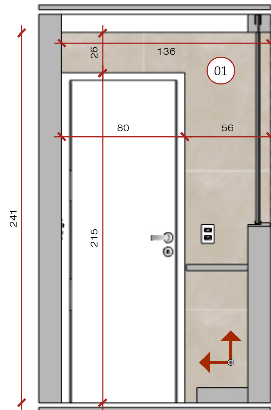
Vista H - Área de Serviço - Paginação Esc: 1/25
