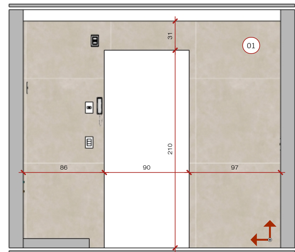
Vista B - Cozinha - Paginação Esc: 1/25
