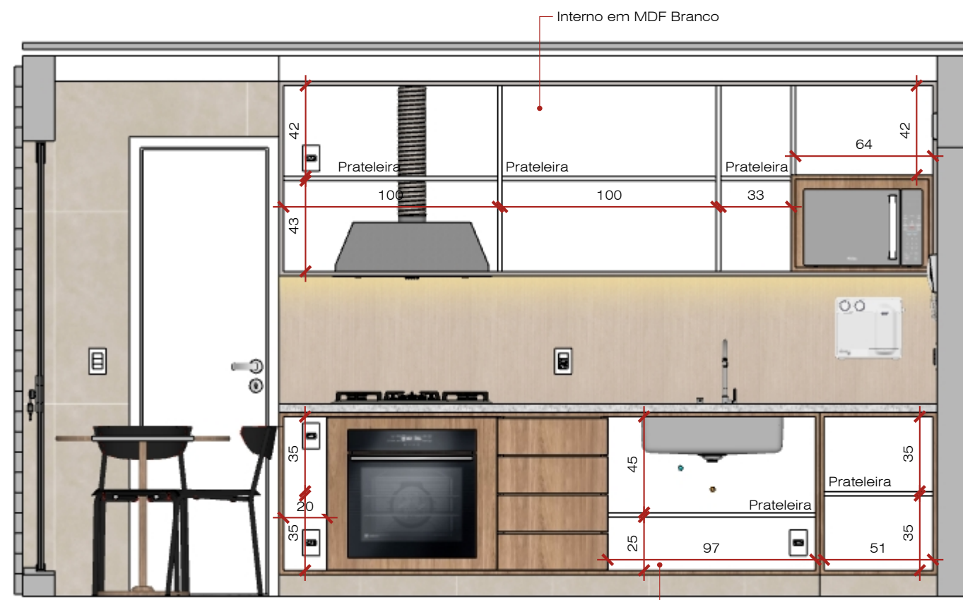
Vista A - Cozinha - Marcenaria Interna Esc: 1/25
