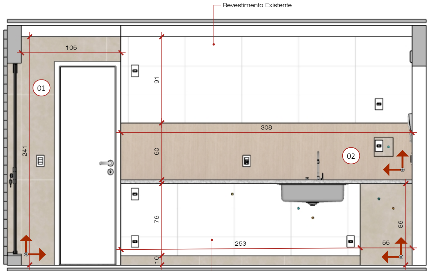
Vista A - Cozinha - Paginação Esc: 1/25
