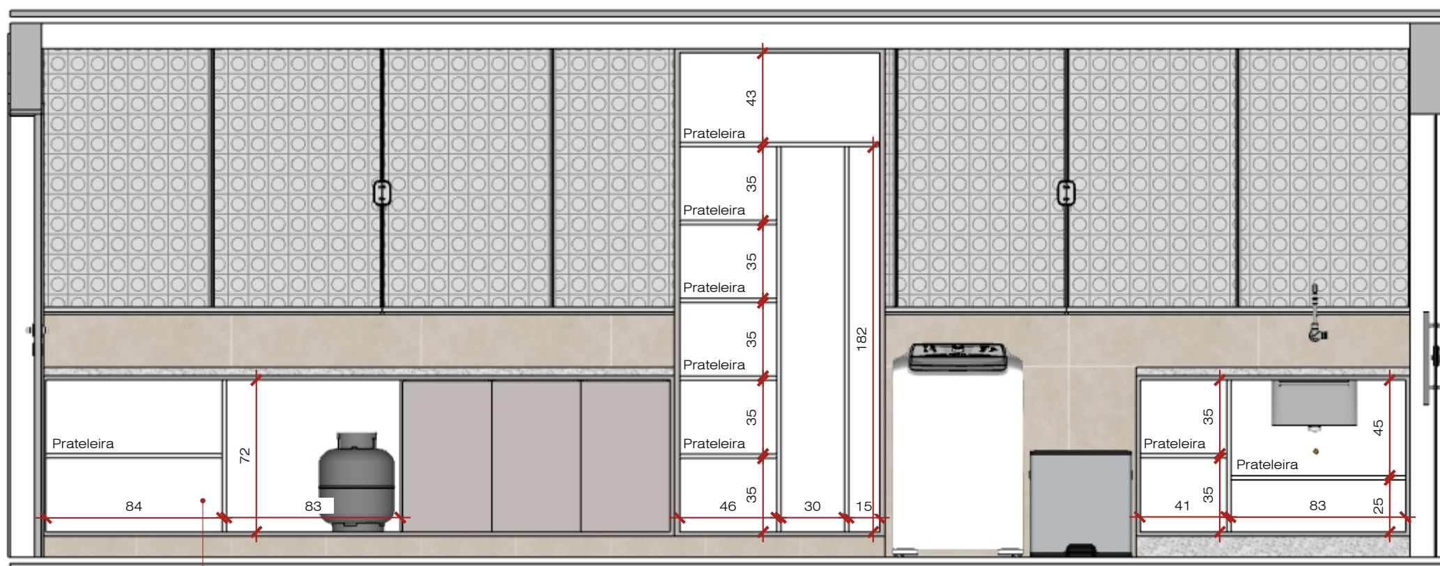
Vista E - Área de Serviço - Marcenaria Interna Esc: 1/25
