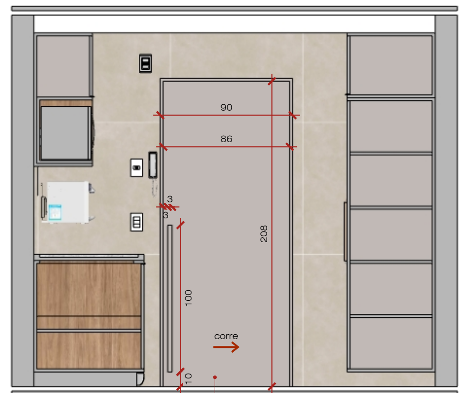
Vista B - Cozinha - Marcenaria Esc: 1/25
