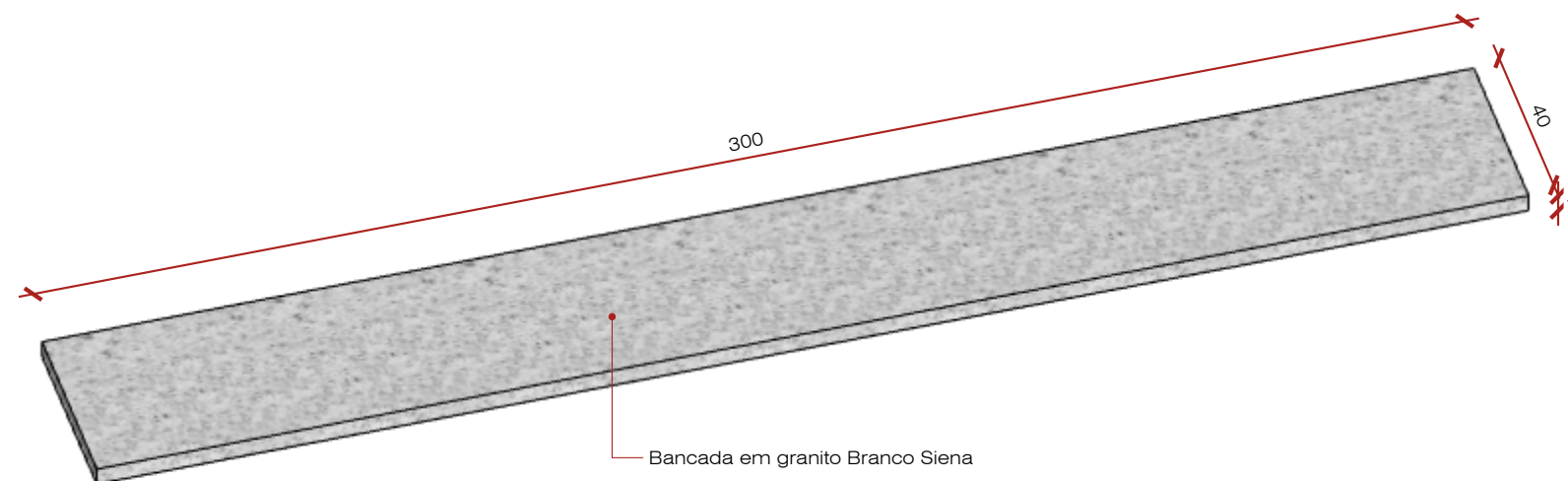
Vista E - Área de Serviço - Marmoraria Esc: 1/15
