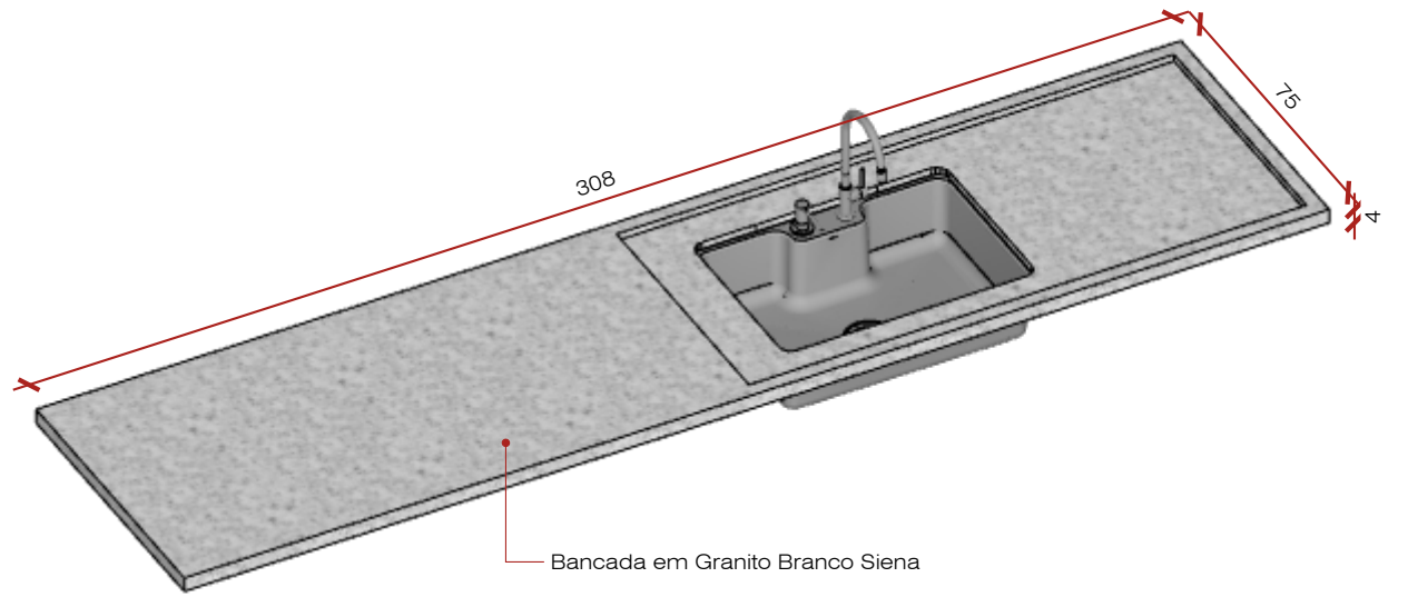
Vista A - Detalhe - Marmoraria Esc: 1/25
