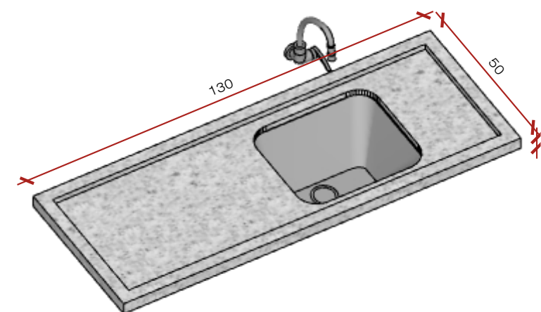
Vista E - Área de Serviço - Marmoraria Esc: 1/15
