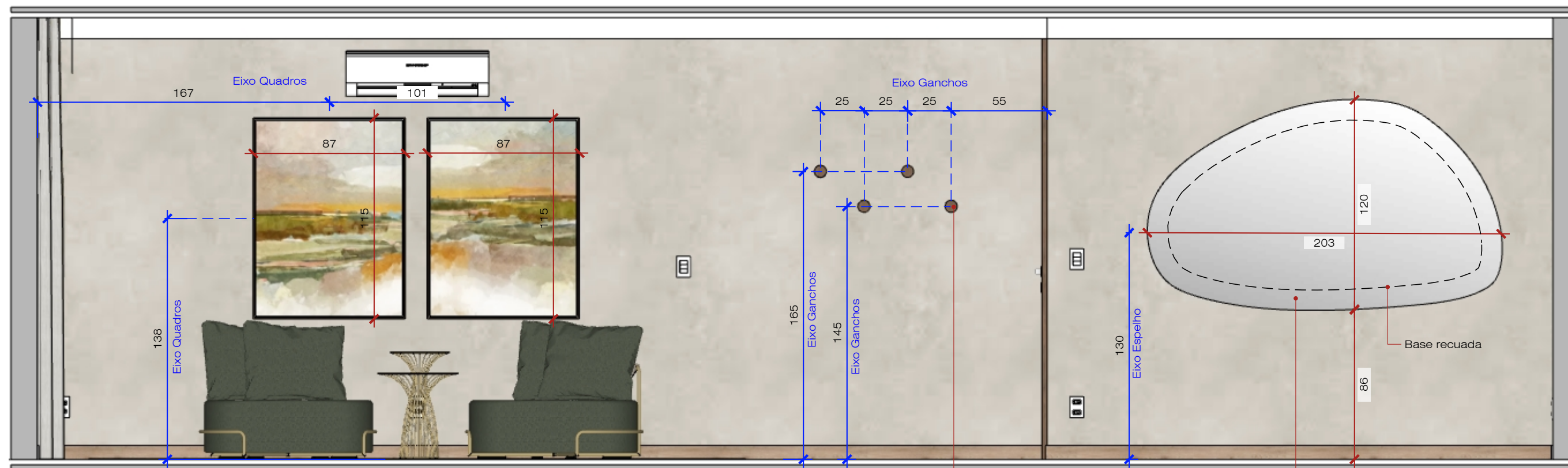
Vista C - Externo Esc: 1/25
