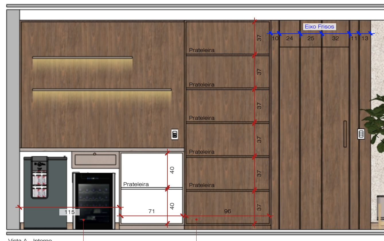
Vista A - Interno Esc: 1/25
