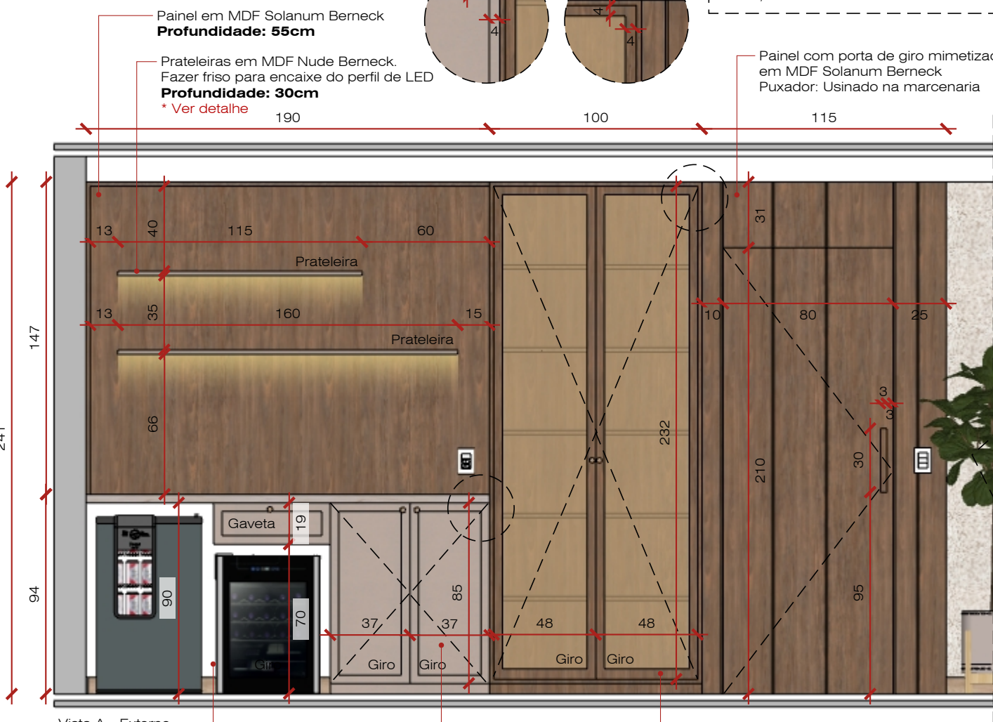
Vista A - Externo Esc: 1/25
