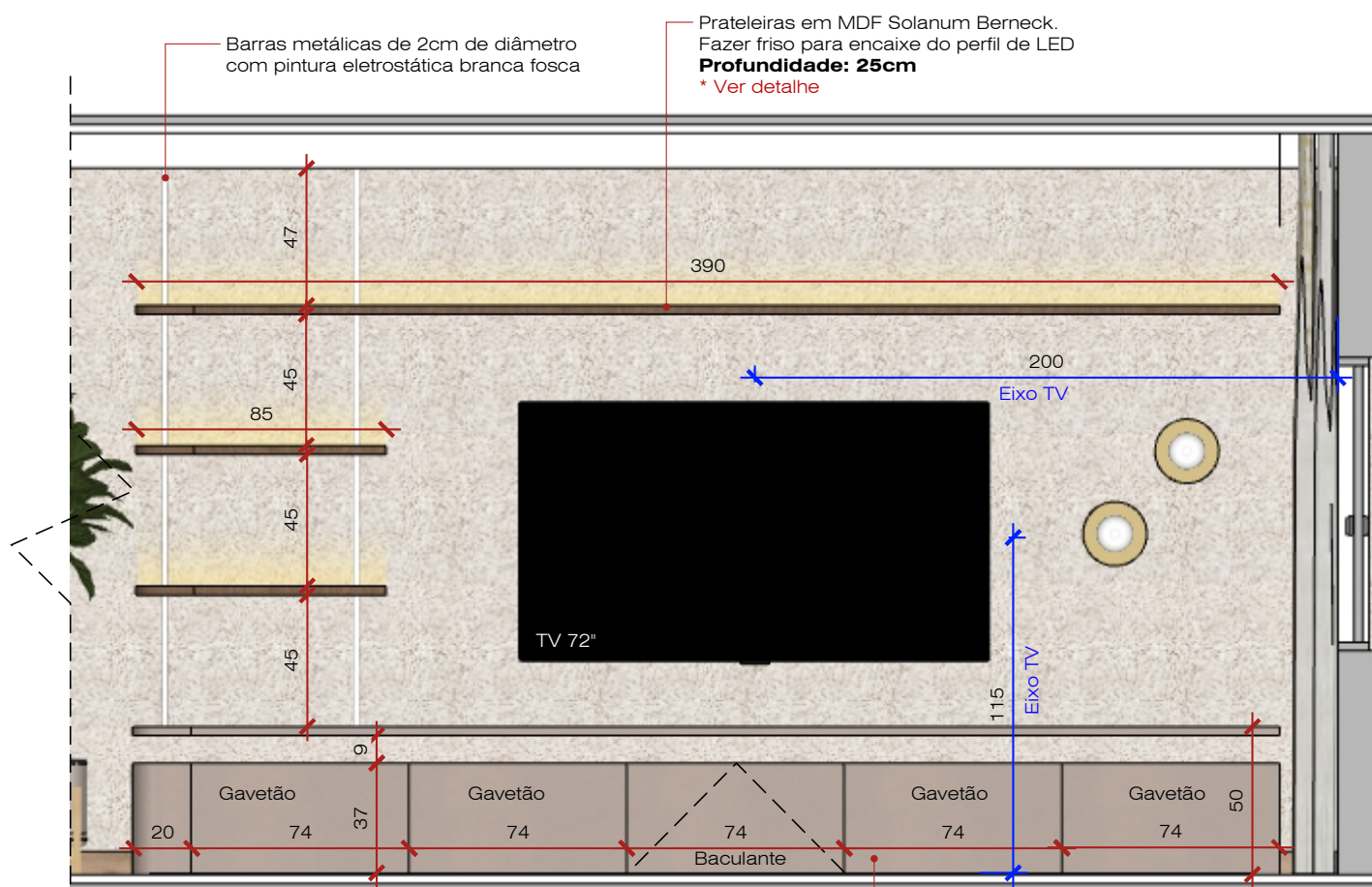
Vista A - Externo Esc: 1/25
