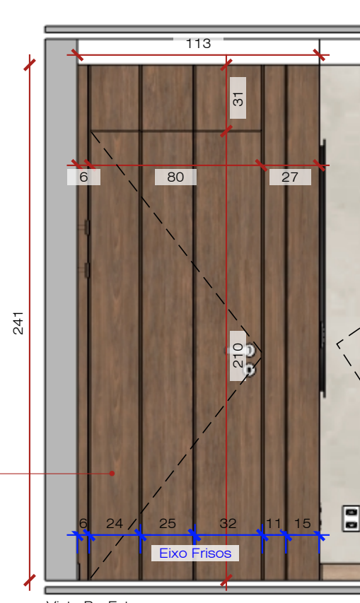
Vista B - Externo Esc: 1/20
