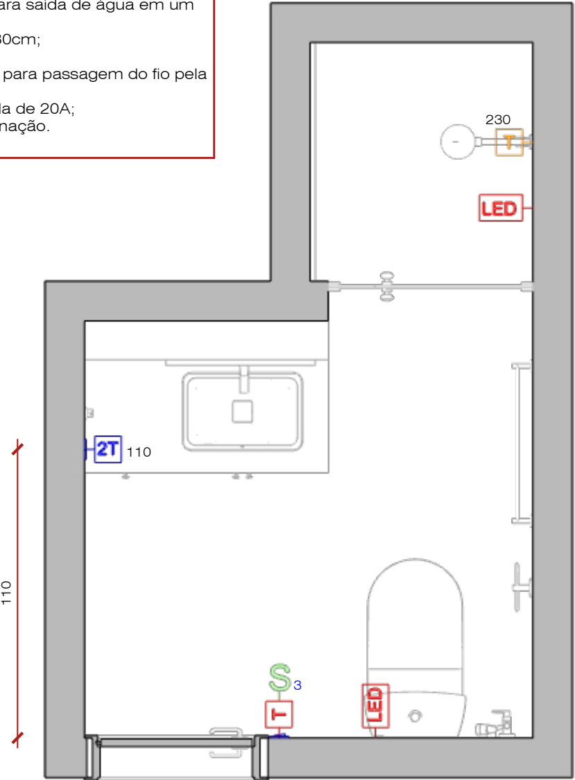
Planta de alteração dos pontos elétricos Esc: 1/20
