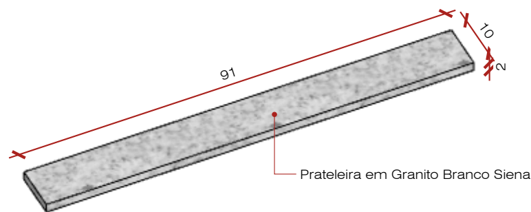
Vista D - Marmoraria Esc: 1/10
