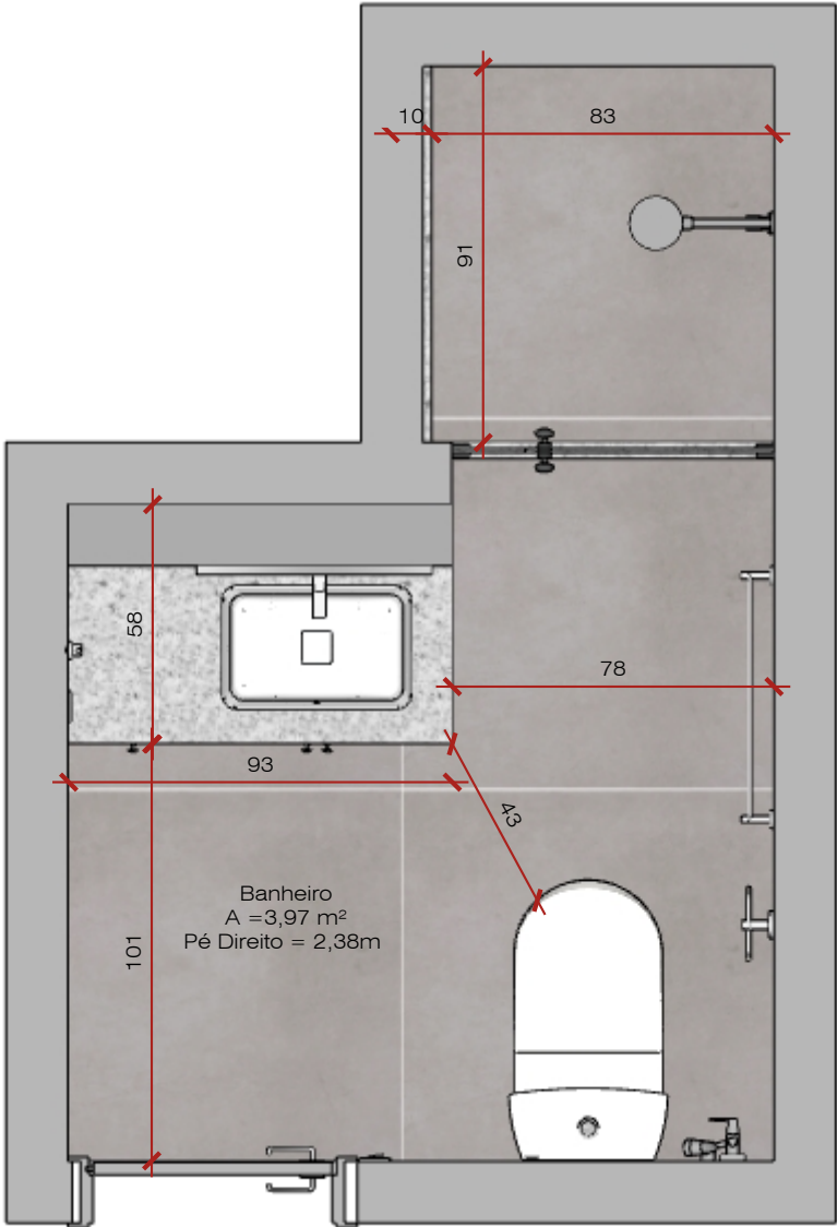
Planta de Layout Esc: 1/20
