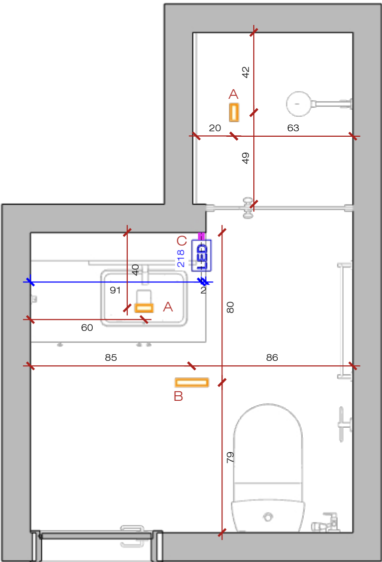
Planta de Iluminação Esc: 1/20
