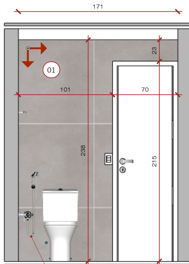
Vista C - Paginação Esc: 1/25 Instalar ducha de forma que o acabamento fique alinhado com o ponto da água e o rabicho não encoste no chão
