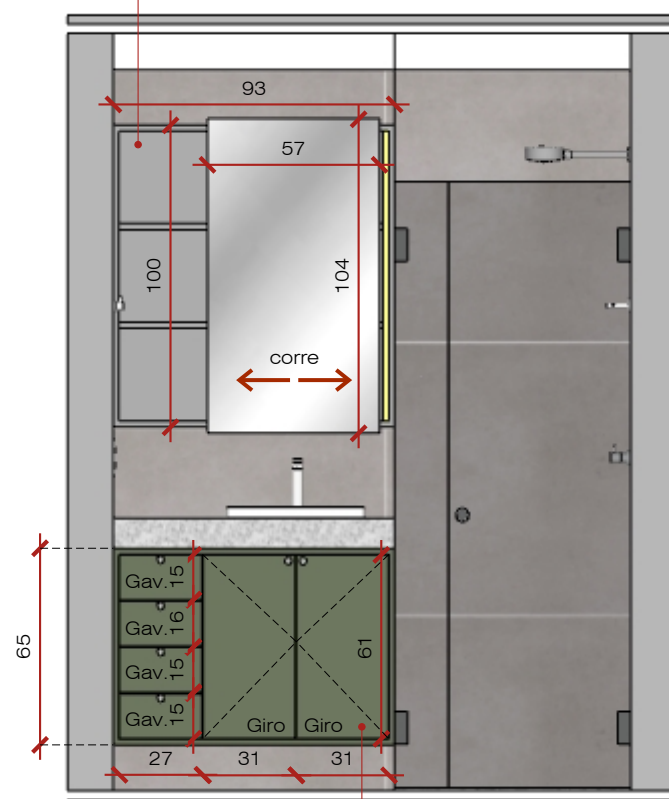
Vista A - Marcenaria Externa Esc: 1/25
