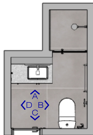
Planta Baixa Esc: 1/50
