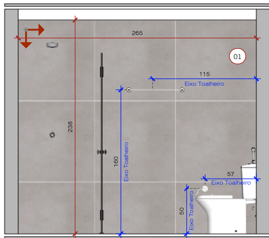
Vista B - Paginação Esc: 1/25
