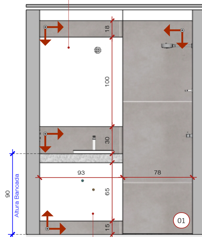
Vista A - Paginação Esc: 1/25
