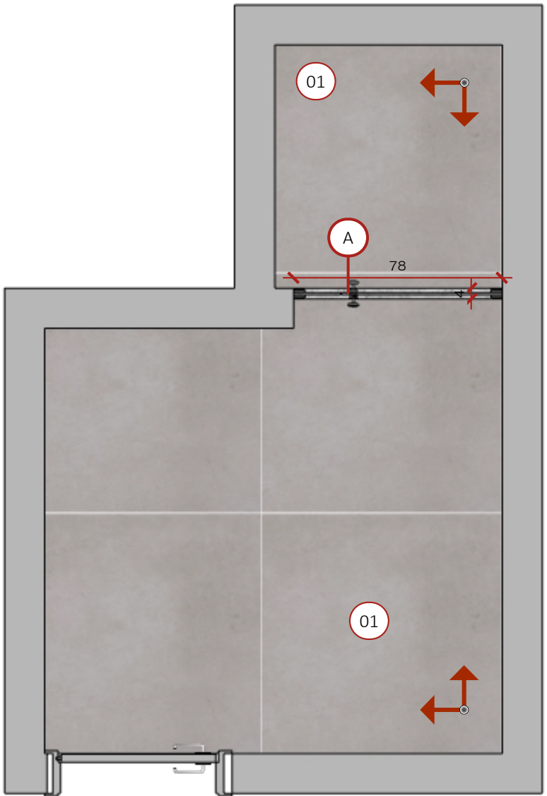
Planta de Paginação de Piso Esc: 1/20
