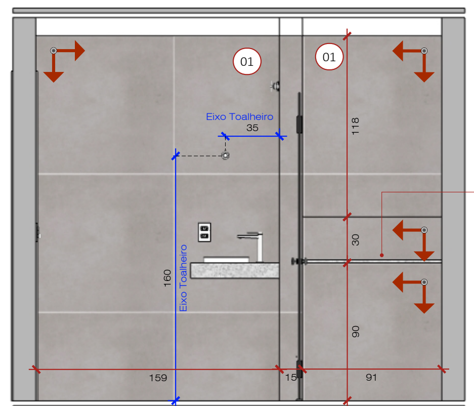
Vista D - Paginação Esc: 1/25
