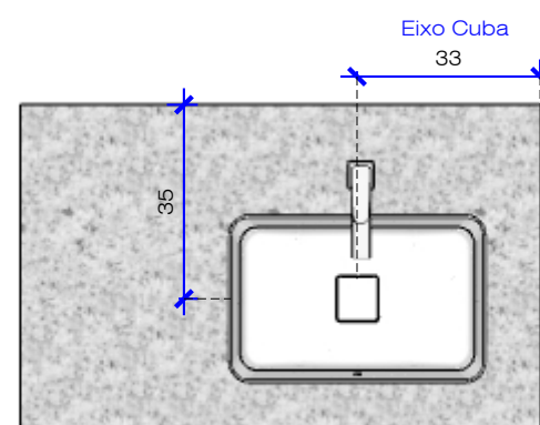
Vista A - Marmoraria - Detalhe Esc: 1/15
