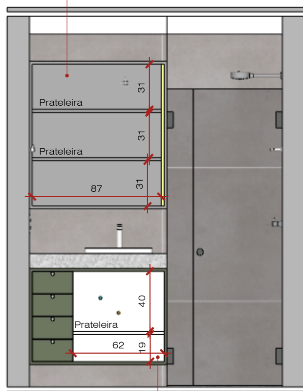
Vista A - Marcenaria Interna Esc: 1/25
