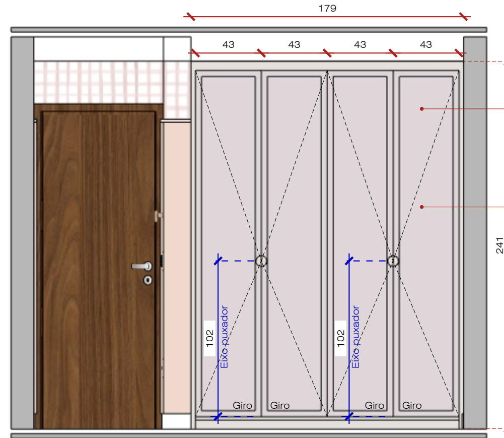
Vista A - Marcenaria Esc: 1/25
