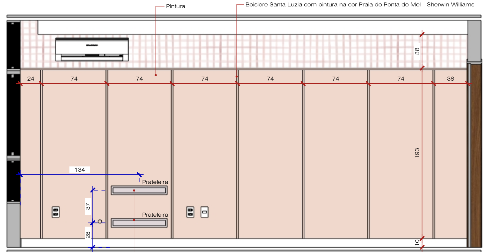
Vista B - Boisiere Esc: 1/25
