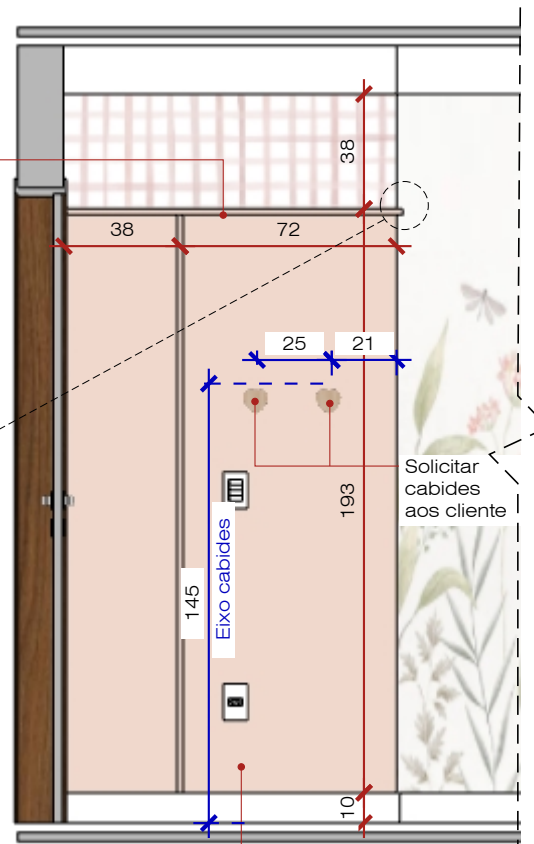
Vista C - Boisiere Esc: 1/25
