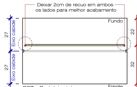
DET - Prateleira interna Esc: 1/15
