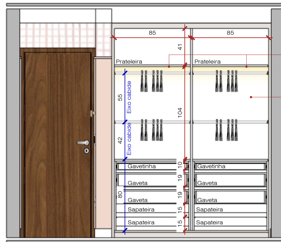
Vista A - Marcenaria interna Esc: 1/25
