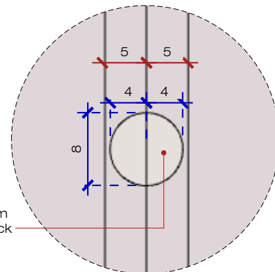
DET - Puxador cava roupeiro Esc: 1/5
