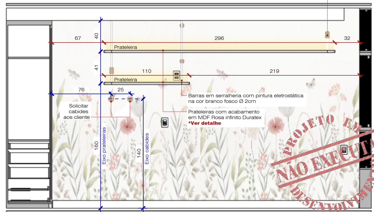
Vista D - Marcenaria e Paginação Esc: 1/25
