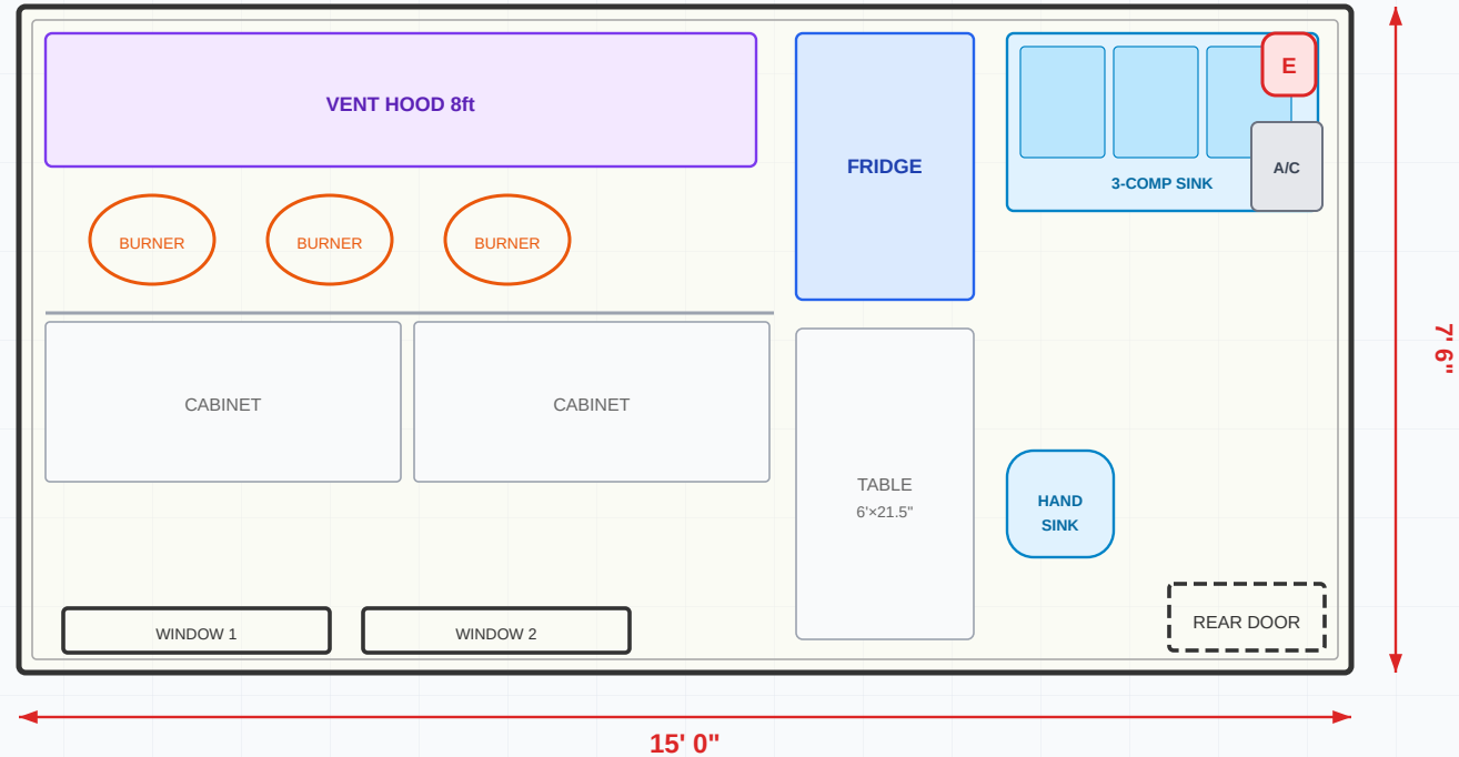
TOP VIEW / PLANTA
