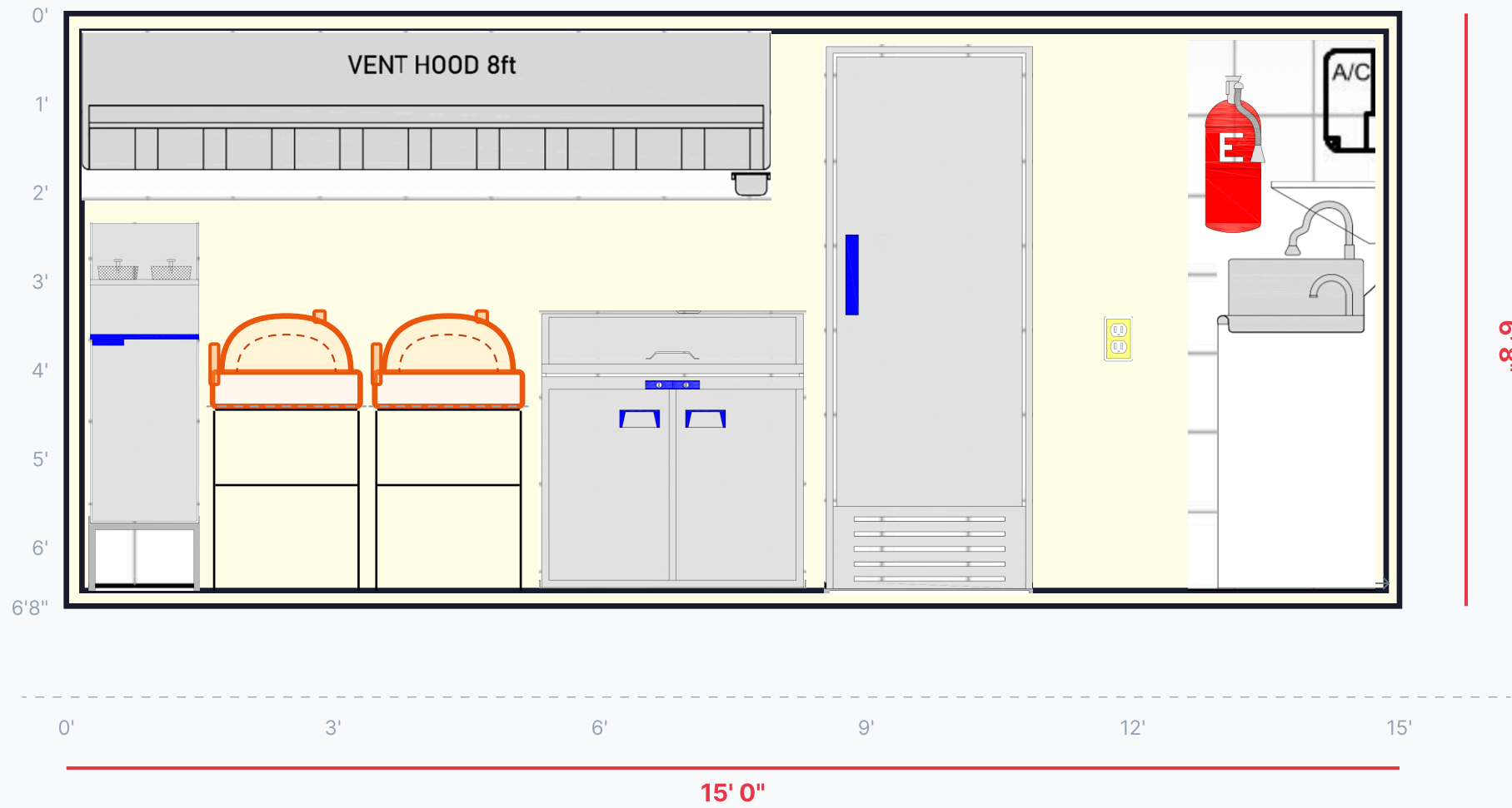
RIGHT SIDE VIEW (LADO DERECHO)
