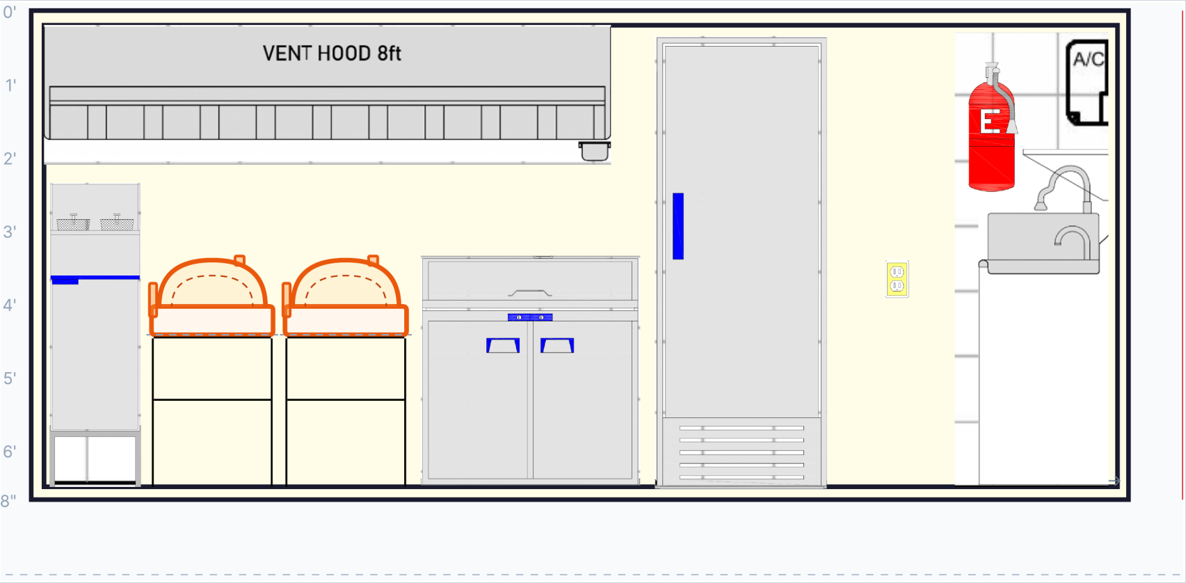
LEFT SIDE VIEW (LADO IZQUIERDO)
