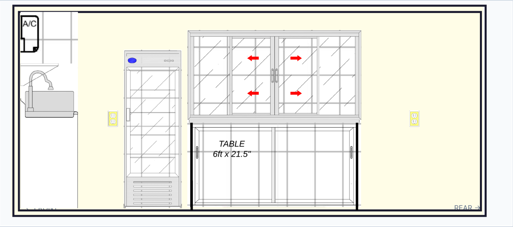
RIGHT SIDE VIEW (LADO DERECHO)
