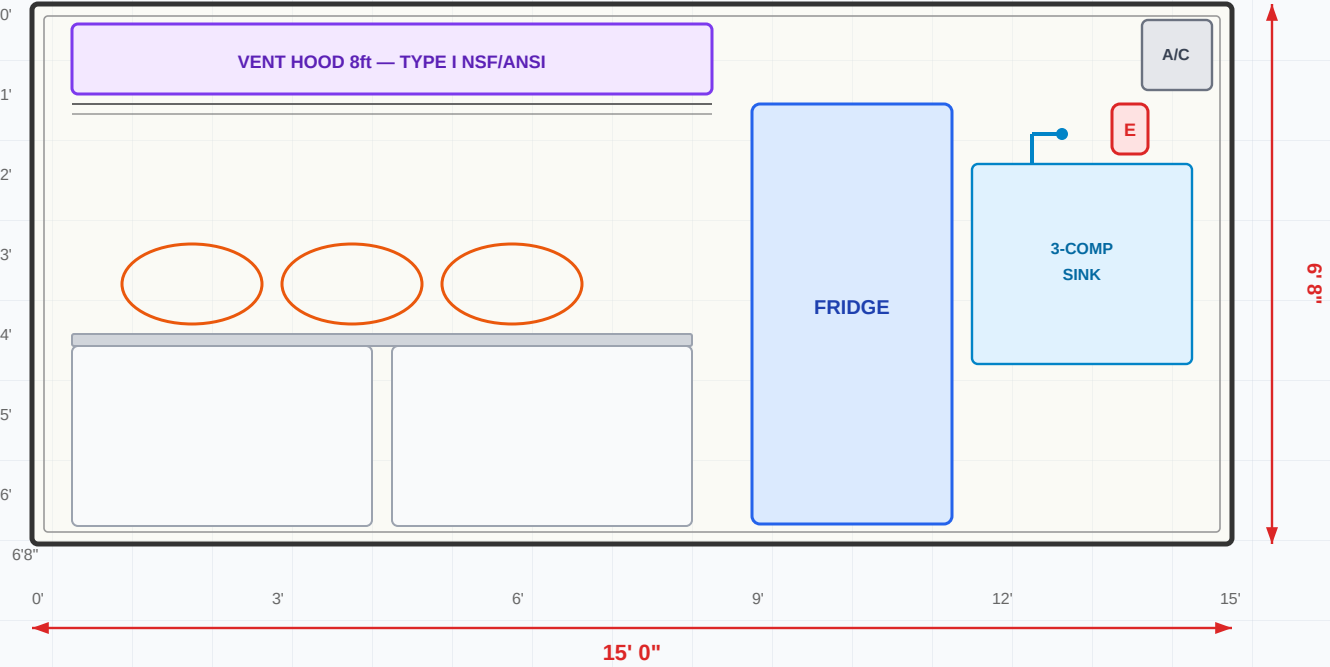
RIGHT SIDE VIEW (LADO DERECHO)
