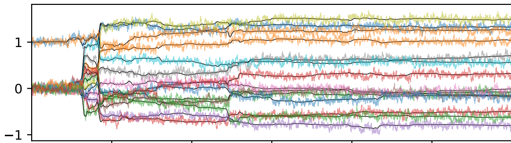
Parameter dynamics
