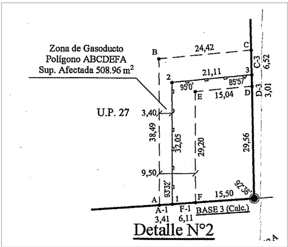
Polígono ABCDEFA, 508,96 m² afectados dentro de la U.P. 27, sobre el sector de Calle 8. Servidumbre a favor de Naturgy BAN S.A.
